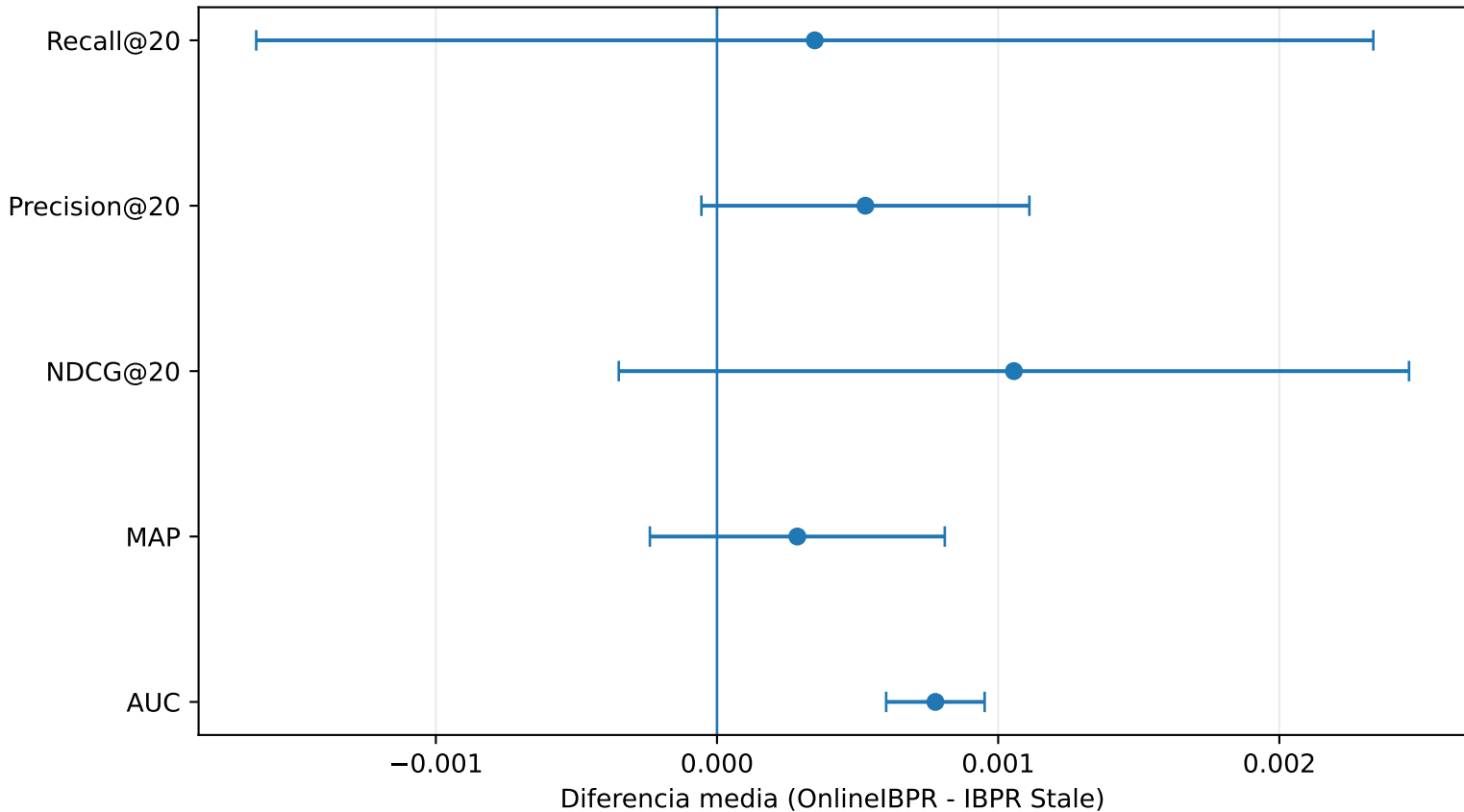
Deltas emparejados en el holdout final con intervalo de confianza del 95%
