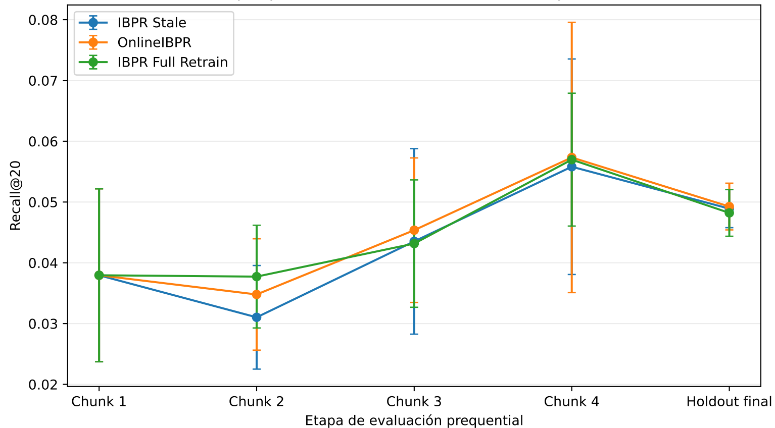
Evolución prequential de Recall@20 durante el flujo incremental
