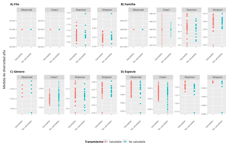
Figura 4.10: Diversidad alfa de las bacterias por nivel taxonómico: A) filo, B) familia, C) género, D) especie. (Script)
