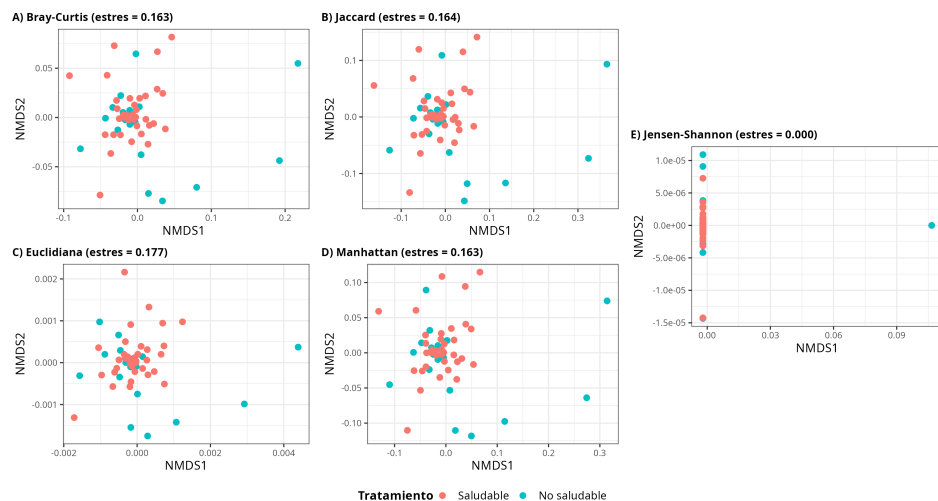
Figura 4.3: Ordenaciones NMDS de la diversidad beta de la comunidad completa para cinco medidas de disimilitud. A) Bray-Curtis. B) Jaccard. C) Euclidiana. D) Manhattan. E) Jensen-Shannon. Ninguna medida separa las muestras saludables de las no saludables. (Script)
