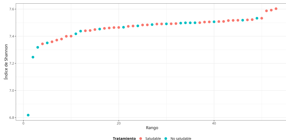
Figura 4.14: Valores del índice de Shannon de la comunidad completa ordenados por rango, coloreados por grupo. Los grupos aparecen mezclados en todo el recorrido. Prueba de Wilcoxon-Mann-Whitney: W = 376 , p = 0,259 . (Script)
