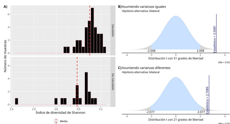
Figura 5. Prueba t de Student sobre el índice de Shannon calculado a nivel de género en eucariotas, grupo que incluye a Fusarium .
