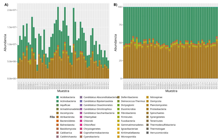
Figura 3. Abundancia de microorganismos a nivel de filo en las 53 muestras analizadas. Nota: A) Abundancia absoluta (número de lecturas asignadas a cada filo). B) Abundancia relativa (porcentaje). Actinobacteria y Proteobacteria dominan la composición taxonómica del conjunto completo de datos. Elaboración propia a partir de datos de Solena Ag.
