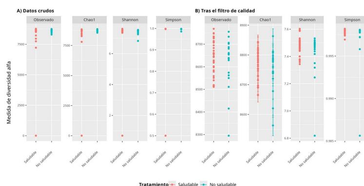
Figura 1. Diversidad alfa (riqueza observada, Chao1, Shannon y Simpson) en muestras saludables y no saludables.
