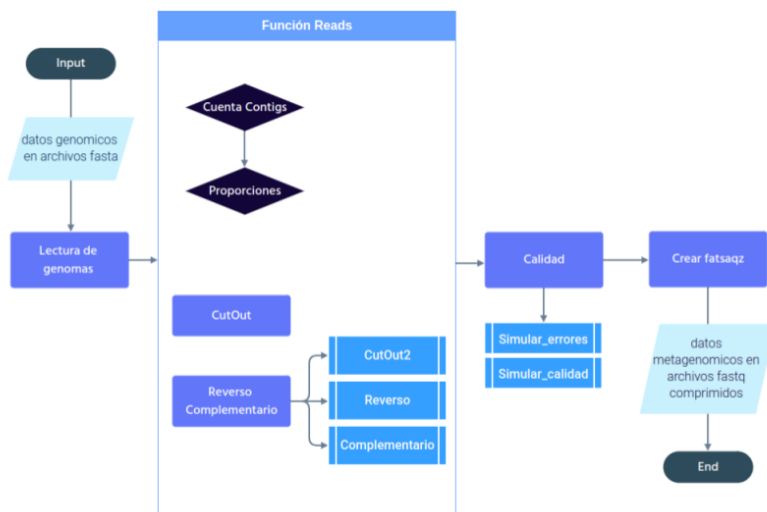
Figura 3.2: Diagrama de Flujo PyMetaSeem
