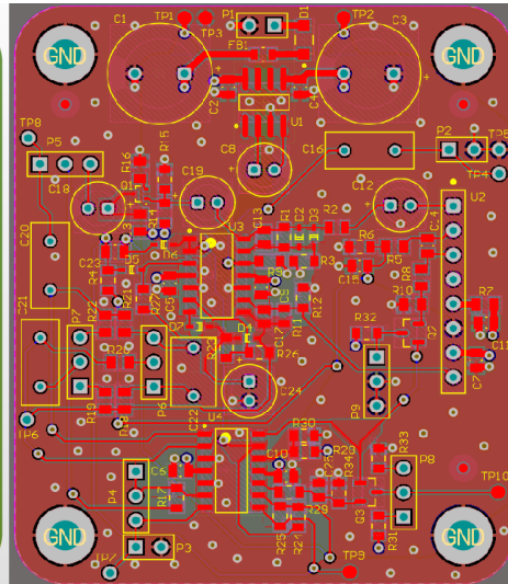
Altium PCB/Layout
