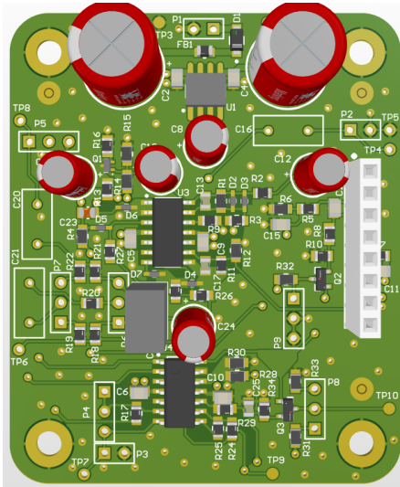
Altium PCB/Layout
