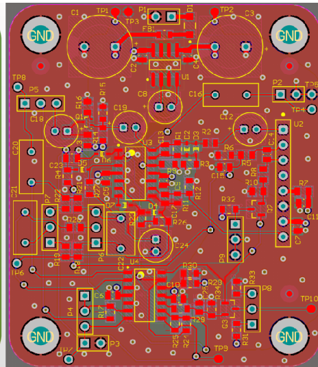
Altium PCB/Layout
