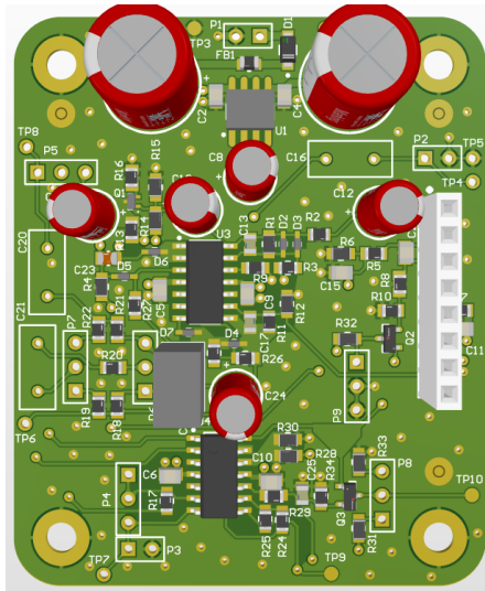
Altium PCB/Layout
