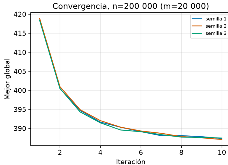
Figura 5: Convergencia (mejor global vs. iteración), n=200 000, m=20 000, 3 semillas.
