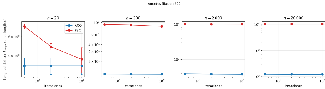
Figura 7: L_{mejor} contra iteraciones, con 500 agentes.
