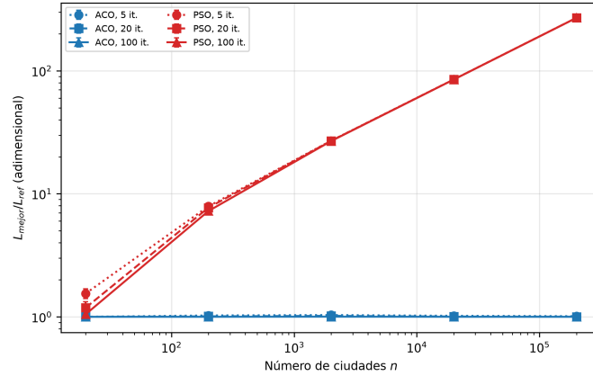
Figura 9: L_{mejor}/L_{ref} contra n con 2 048 agentes ( L_{ref} : óptimo de Held-Karp en n = 20 ; en los demás n , la mejor longitud medida).
