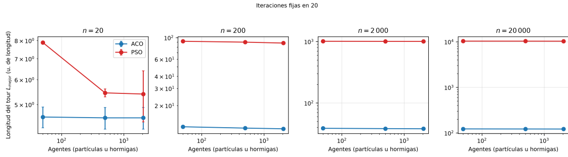
Figura 6: L_{mejor} contra agentes, con 20 iteraciones.
