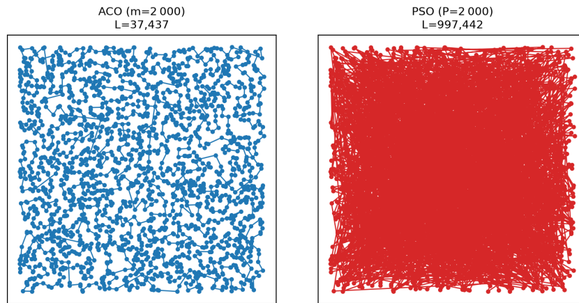
Figura 11: Rutas en n = 2000 : ACO y PSO (semilla 1, 50 iteraciones).
