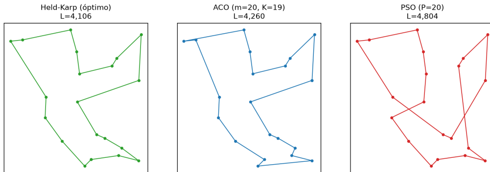
Figura 10: Rutas en n = 20 : óptimo de Held-Karp, ACO y PSO (semilla 1, 100 iteraciones).
