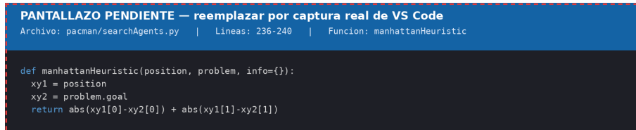
Figura 3: manhattanHeuristic en pacman/searchAgents.py (líneas 236-240).
