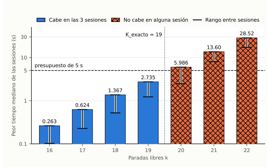
Figura 8: Medición de Held-Karp en esta máquina: peor tiempo mediano de las sesiones contra k , con el presupuesto de 5 s y K_{\text{exacto}} . Fuente: elaboración propia
