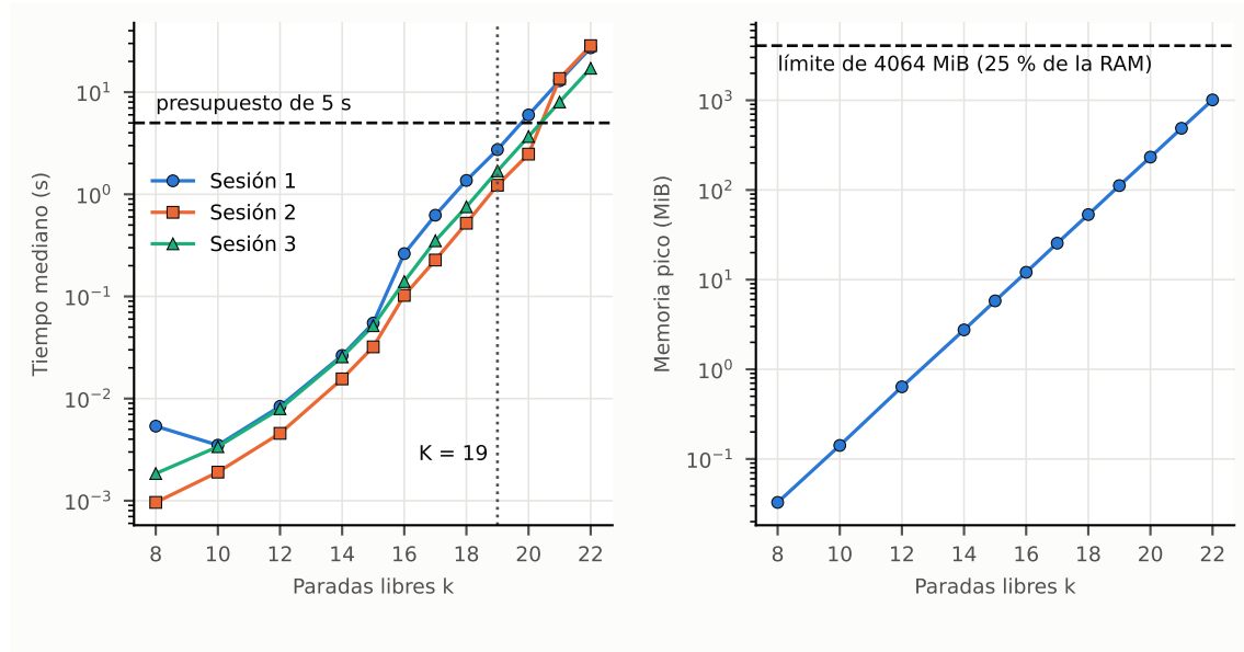
Figura 8: Medición de Held-Karp en esta máquina: tiempo mediano por sesión y memoria pico contra k , con el presupuesto de 5 s, el límite de memoria y K_{\text{exacto}} . Fuente: elaboración propia
