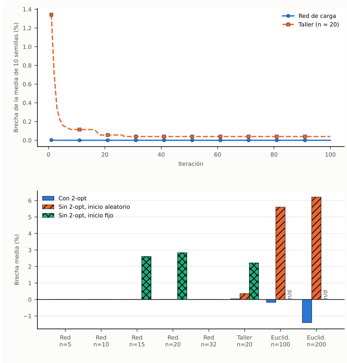
Figura 9: Convergencia del ACO con 2-opt (arriba) y brecha media por grupo con y sin 2-opt (abajo). Fuente: elaboración propia
