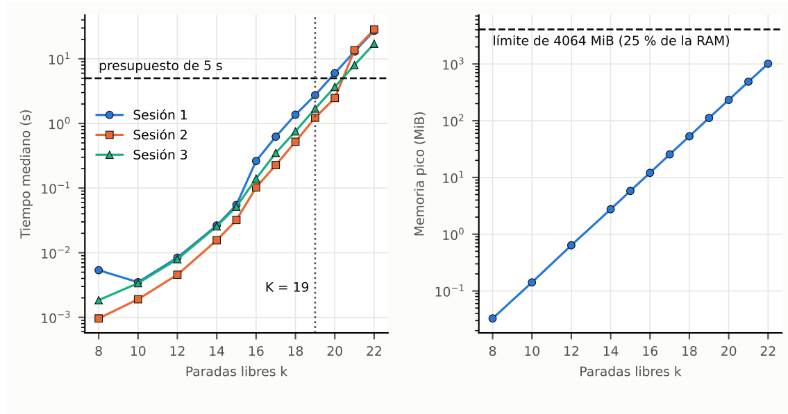
Figura 6: Medición de Held-Karp en esta máquina: tiempo mediano por sesión y memoria pico contra k , con el presupuesto de 5 s, el límite de memoria y K_{\text{exacto}} . Fuente: elaboración propia
