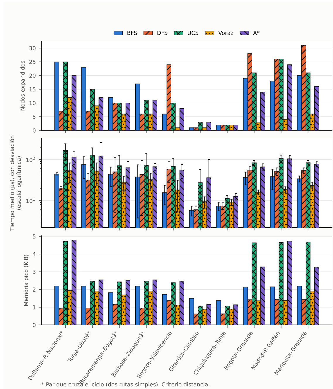
Figura 1: Nodos expandidos, tiempo medio con su desviación y memoria pico de los cinco algoritmos en los diez escenarios, criterio distancia. Fuente: elaboración propia
