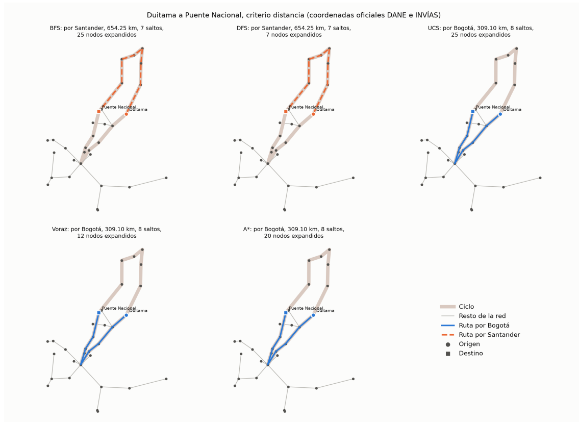
Figura 3: Rutas de los cinco algoritmos, Duitama a Puente Nacional, criterio distancia. Fuente: elaboración propia con datos de INVÍAS y DANE
