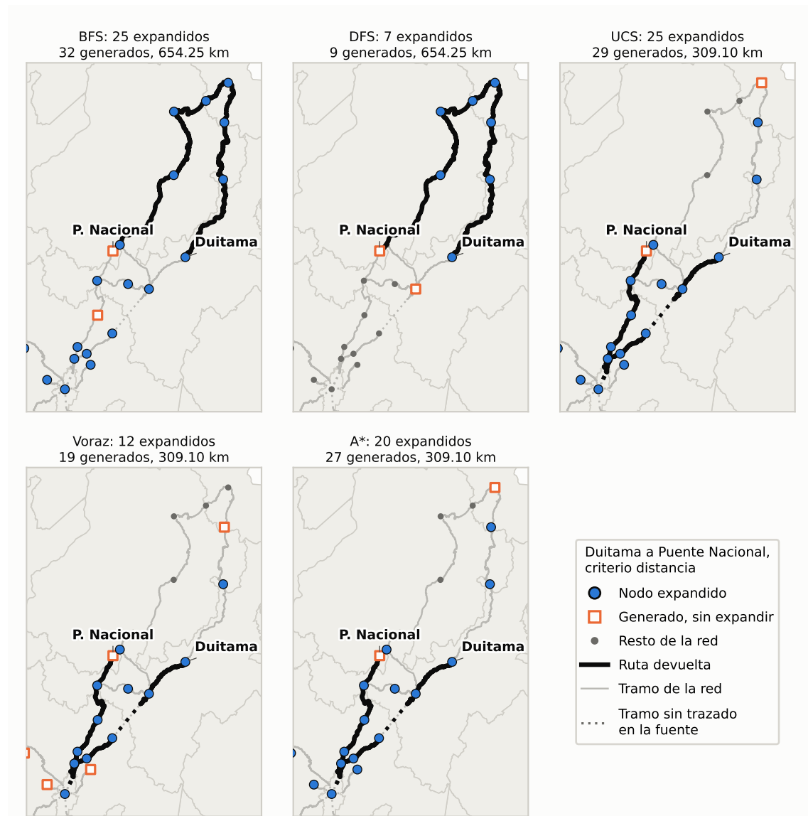
Figura 2: Nodos expandidos y generados por cada búsqueda en el caso central, criterio distancia. Fuente: elaboración propia
