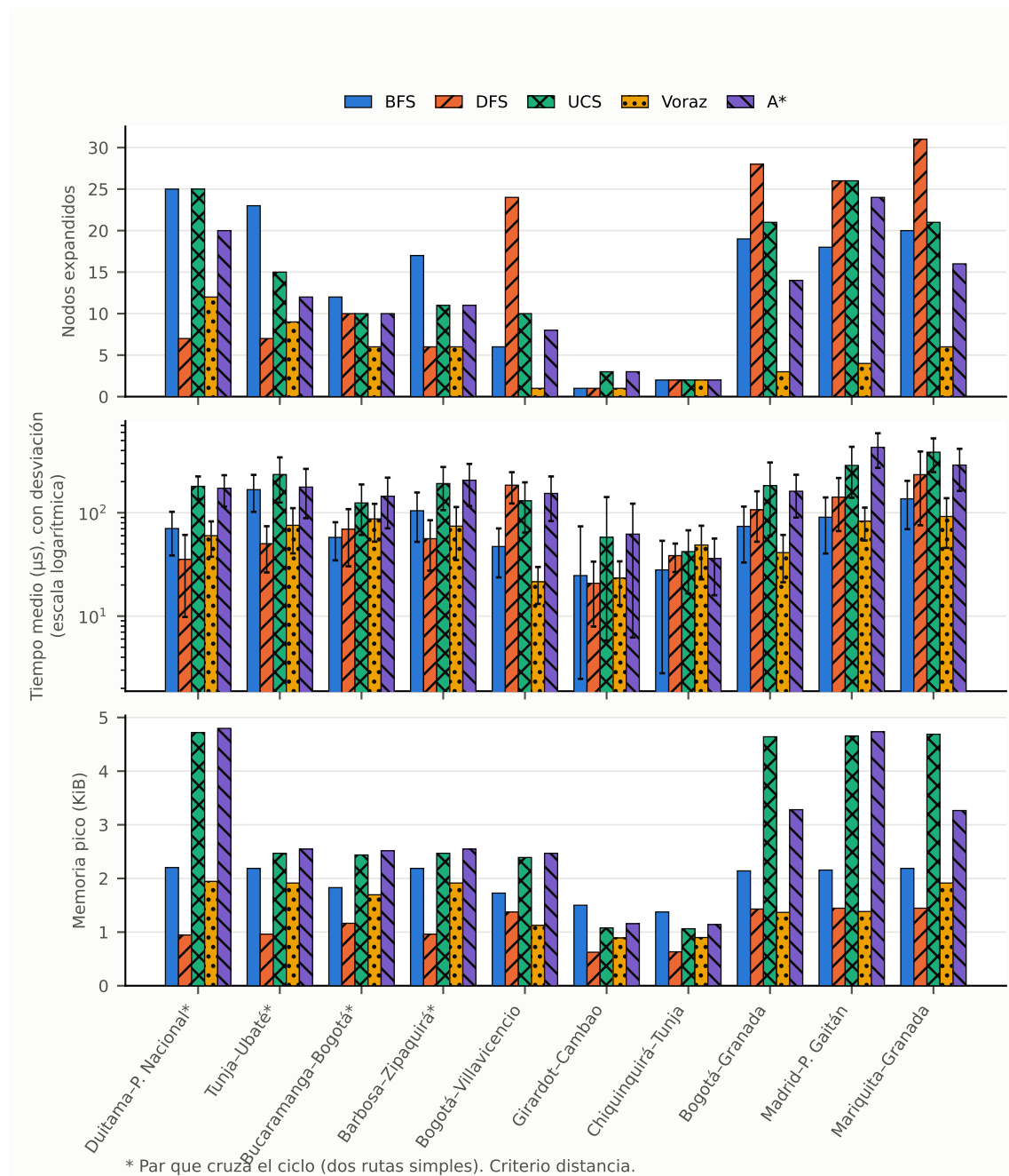
Figura 2: Nodos expandidos, tiempo medio con su desviación y memoria pico de los cinco algoritmos en los diez escenarios, criterio distancia. Fuente: elaboración propia
