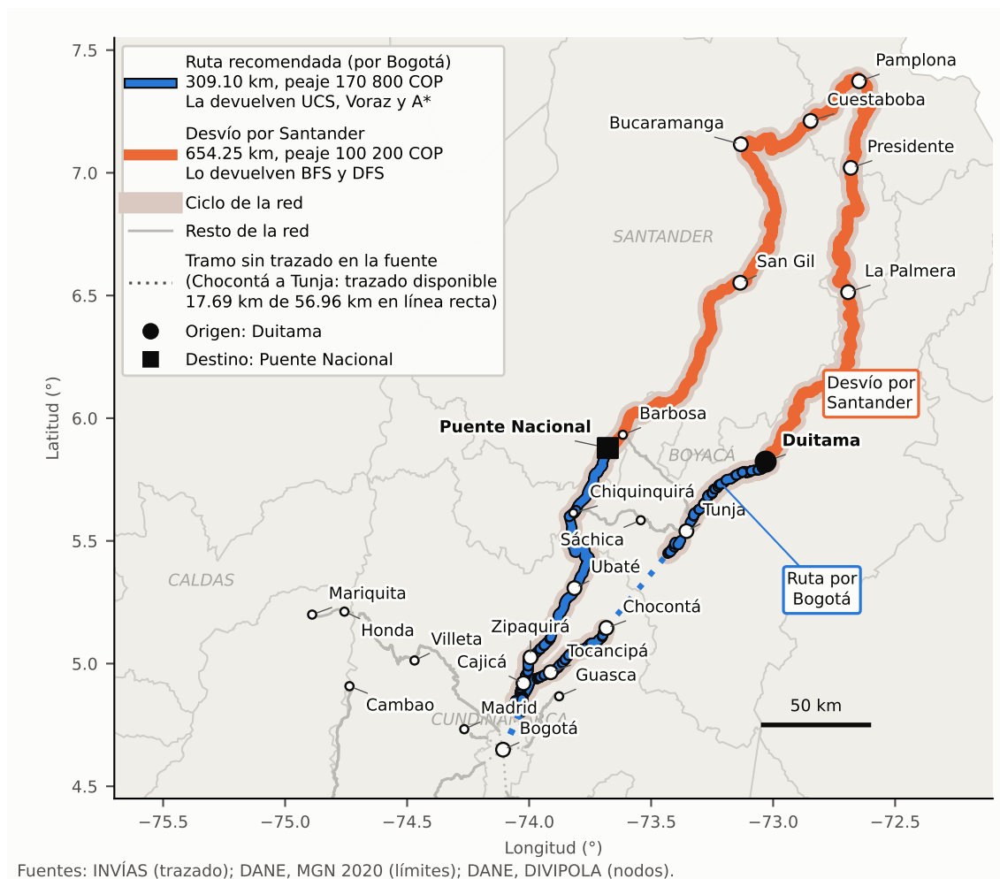
Figura 5: Caso central sobre el mapa: ruta por Bogotá y desvío por Santander. Fuente: elaboración propia con el trazado de INVÍAS, los límites departamentales del DANE [7] y las coordenadas DIVIPOLA
