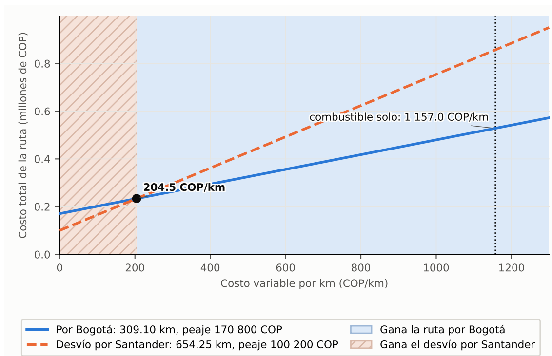
Figura 6: Costo total de las dos rutas de Duitama a Puente Nacional según el costo variable por km. Fuente: elaboración propia
