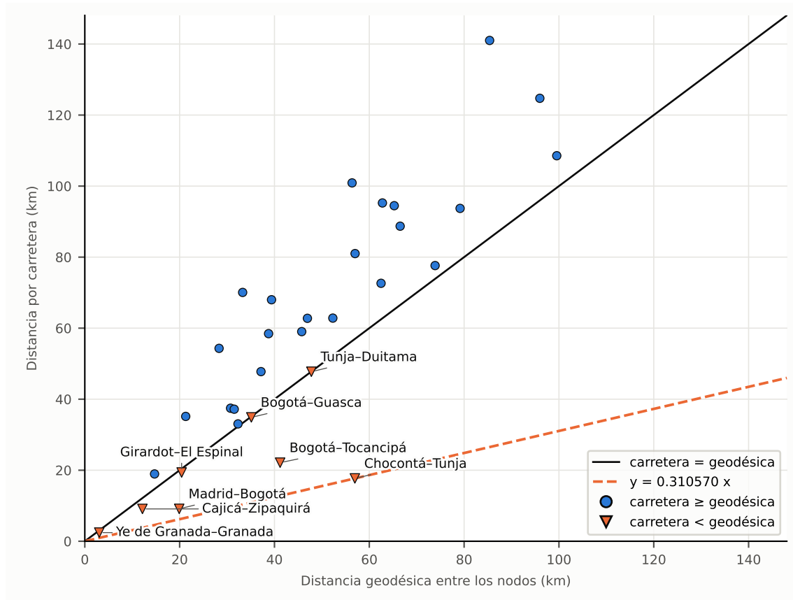
Figura 1: Distancia por carretera contra distancia geodésica de las 32 aristas, con las rectas y = x y y = \alpha x . Fuente: elaboración propia
