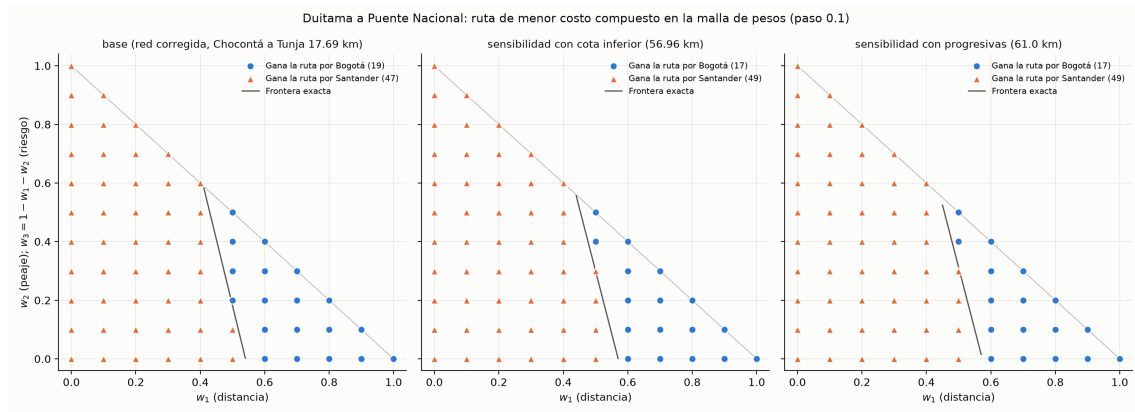
Figura 7: Ruta ganadora en la malla de pesos, con Chocontá a Tunja en 17.69 km (base), en la cota inferior de 56.96 km y en las progresivas de 61.0 km. Fuente: elaboración propia
