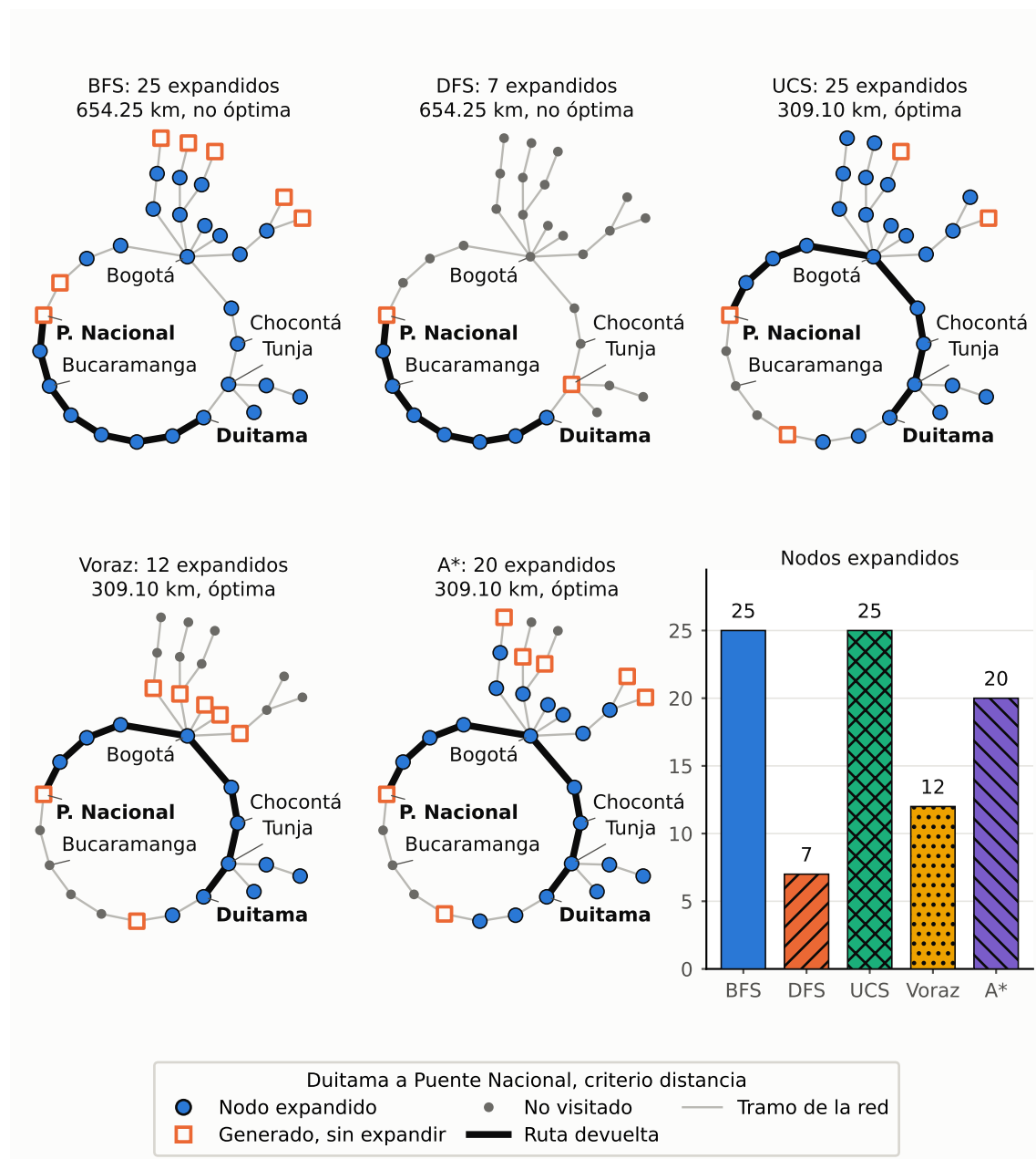
Figura 3: Nodos expandidos, generados sin expandir y no visitados de cada búsqueda en un esquema de la red (el ciclo como anillo), caso central, criterio distancia. Fuente: elaboración propia
