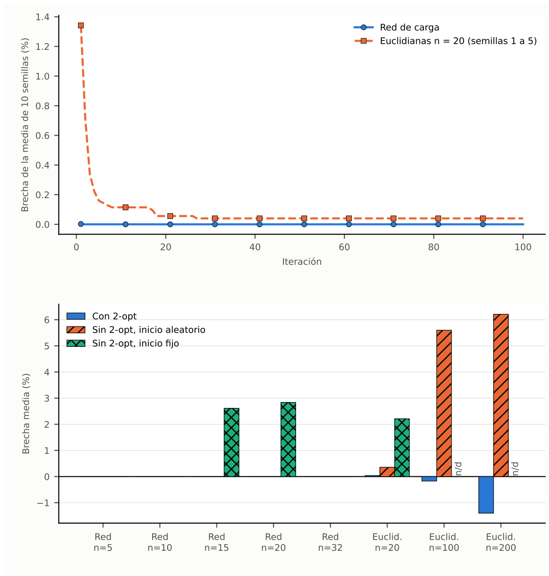
Figura 10: Convergencia del ACO con 2-opt (arriba) y brecha media por grupo con y sin 2-opt (abajo). Fuente: elaboración propia
