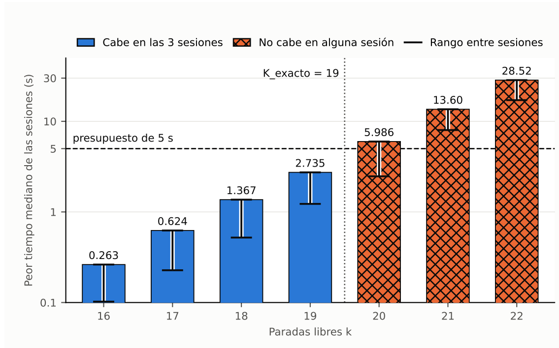
Figura 9: Medición de Held-Karp en esta máquina: peor tiempo mediano de las sesiones contra k , con el presupuesto de 5 s y K_{\text{exacto}} . Fuente: elaboración propia
