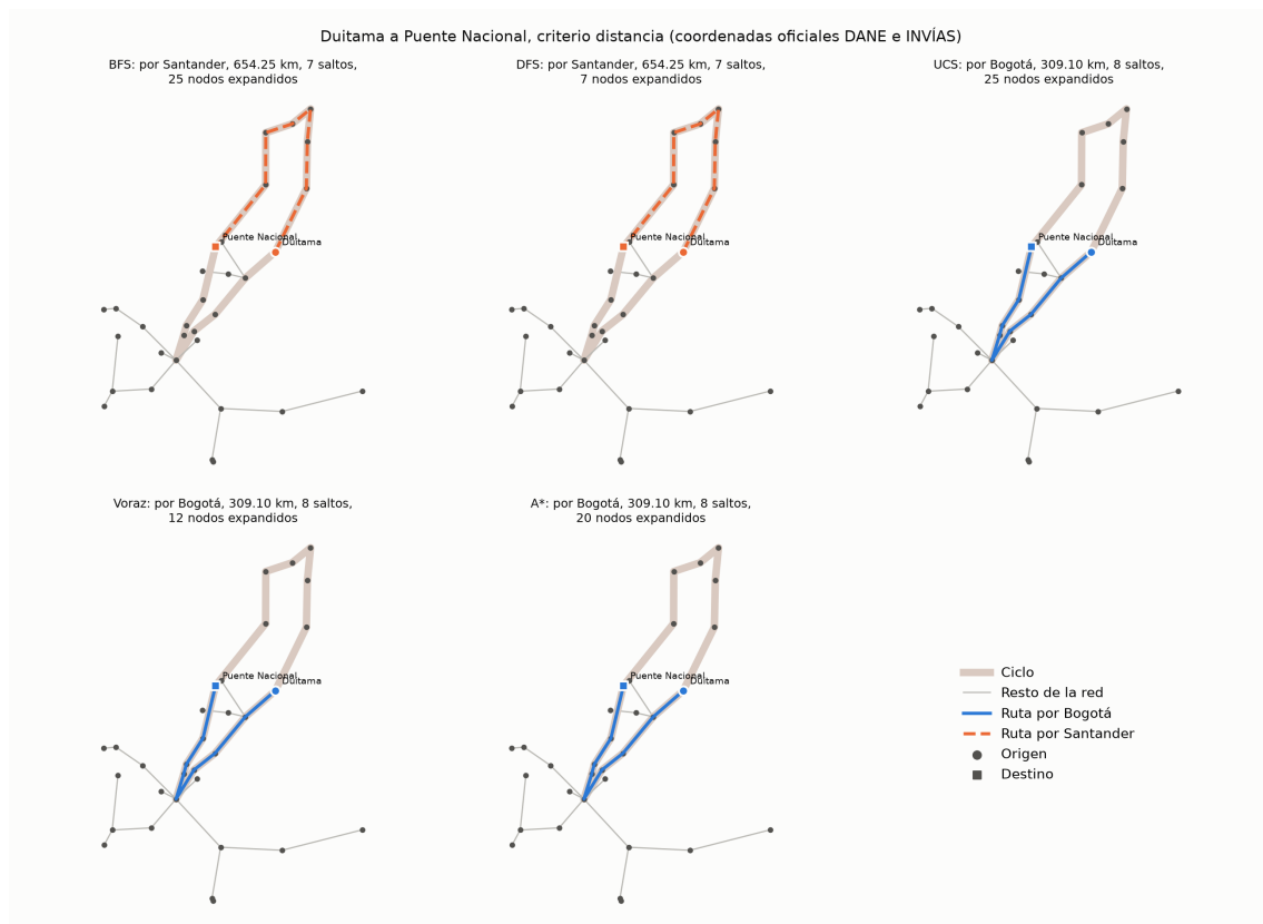
Figura 4: Rutas de los cinco algoritmos, Duitama a Puente Nacional, criterio distancia. Fuente: elaboración propia con datos de INVÍAS y DANE
