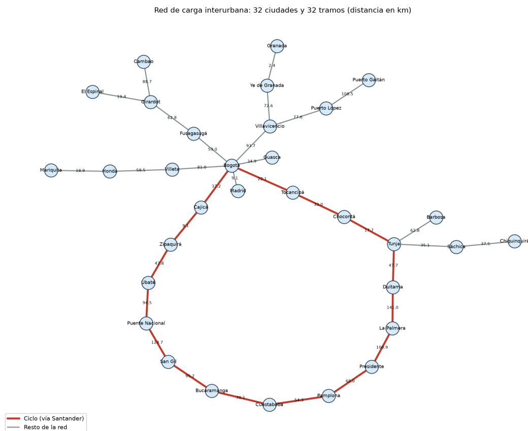
Figura 1: Diagrama de la red de carga. Fuente: elaboración propia
