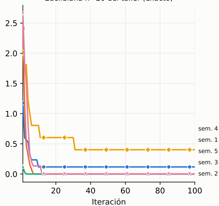
Euclidiana n=20 del taller (exacto)
