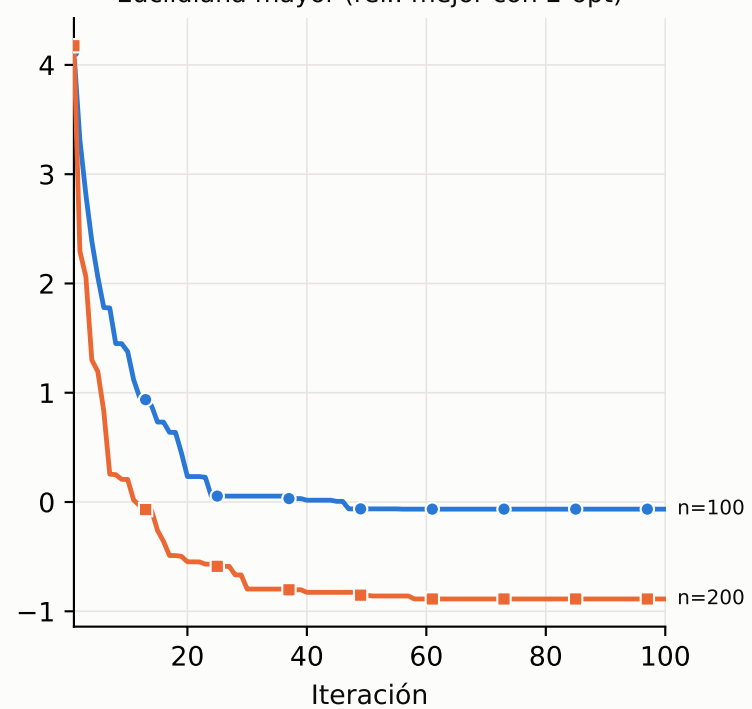
Euclidiana mayor (ref.: mejor con 2-opt)
