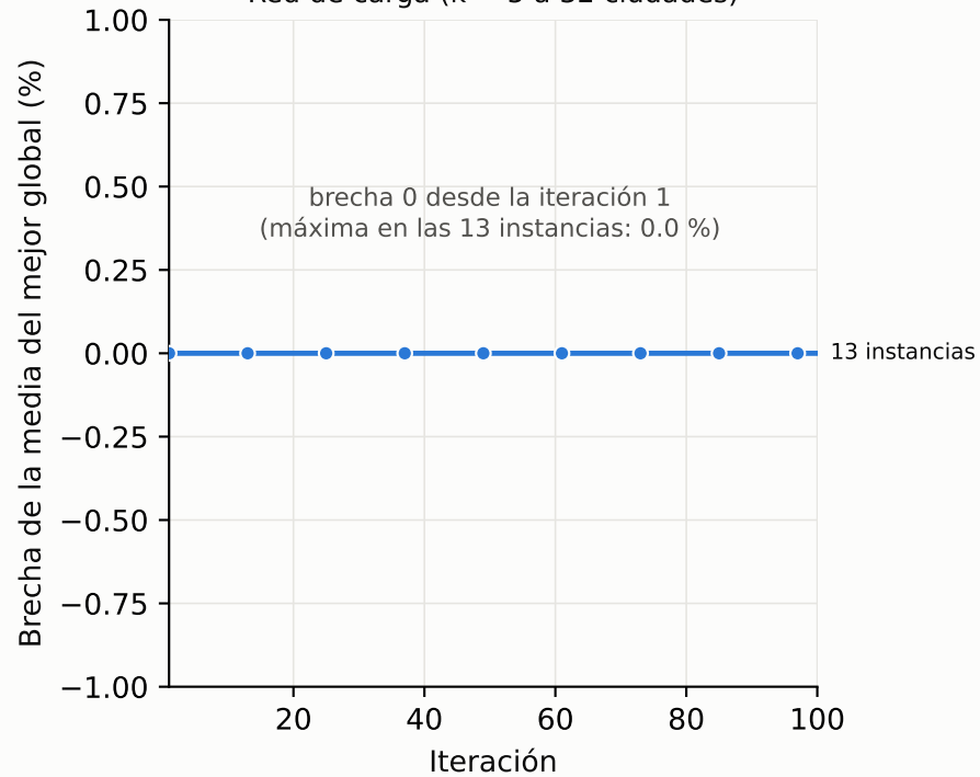
Red de carga (k = 5 a 32 ciudades)
