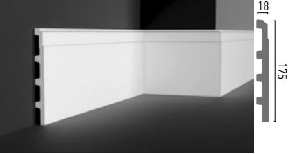
CR 3247 • CR 3247F
