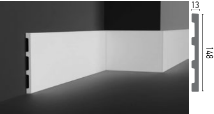
CR 958 • CR 958F
