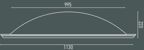
DM 3504 ED: 1130 мм ID: 995 мм D: 220 мм Скловолокно
