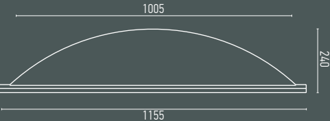
DM 3507 ED: 1155 мм ID: 1005 мм D: 240 мм Скловолокно
