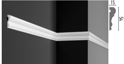
CR 3007 • CR 3007F 54 x 15 мм
