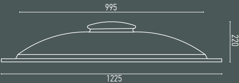
DM 3506 ED: 1225 мм ID: 995 мм D: 220 мм Скловолокно
