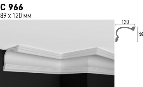
Усі вироби виготовлені з поліуретану F - виріб має гнучкий аналог
