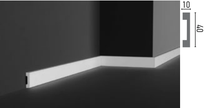
CR 931 • CR 931F
