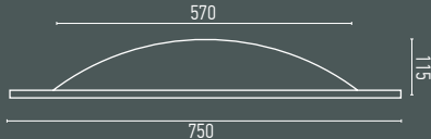
DM 3503 ED: 750 мм ID: 570 мм D: 115 мм Поліуретан
