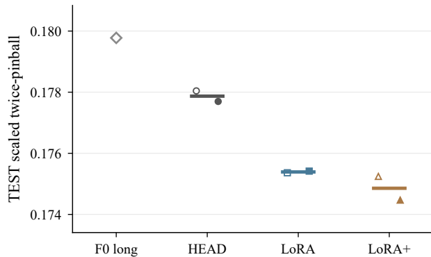
(b) Jena
