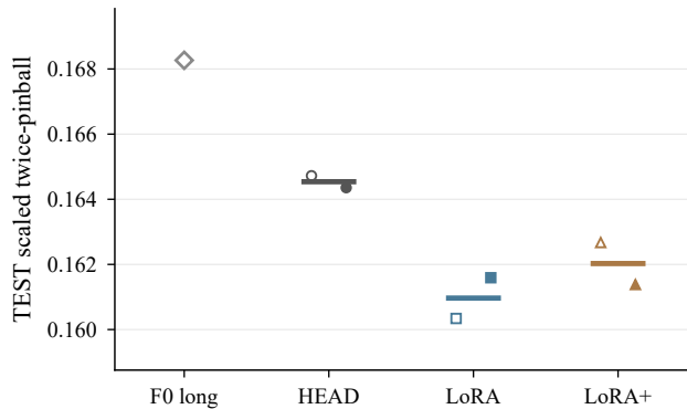
(a) ETTm2
