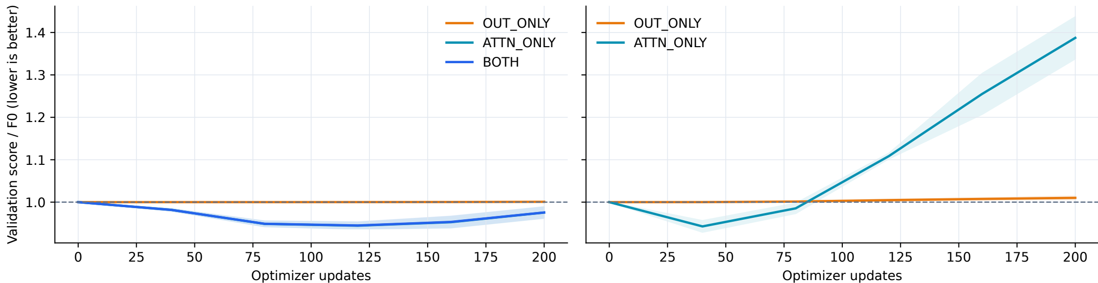
LR 3e-05
