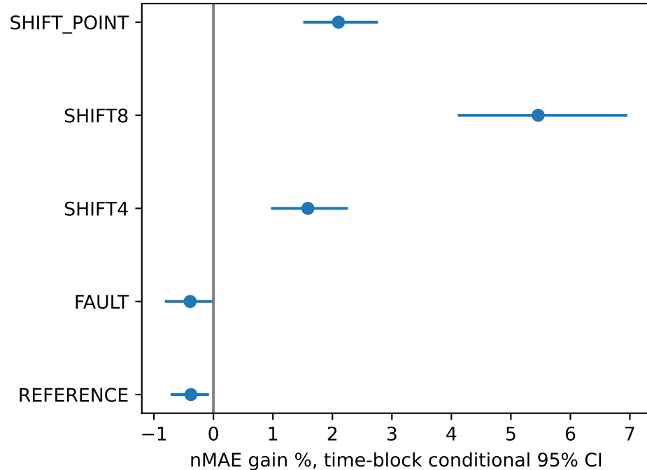
NESO2025: C3 vs C0
