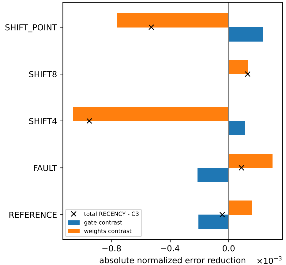
ettm1
