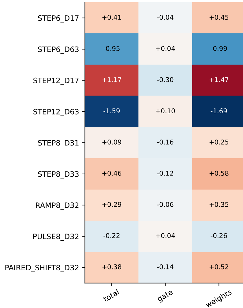
ETTm1
