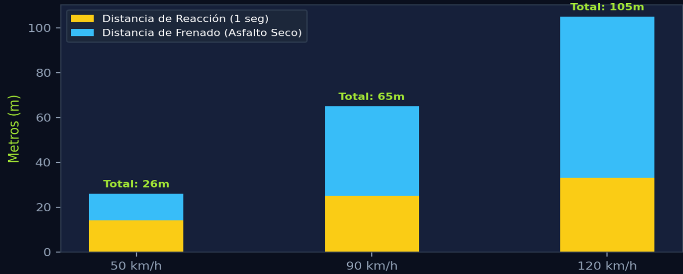
Tema 6: Distancia Total de Detención según la Velocidad en Moto
