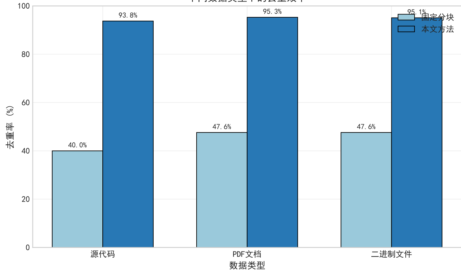
不同数据类型下的去重效率
