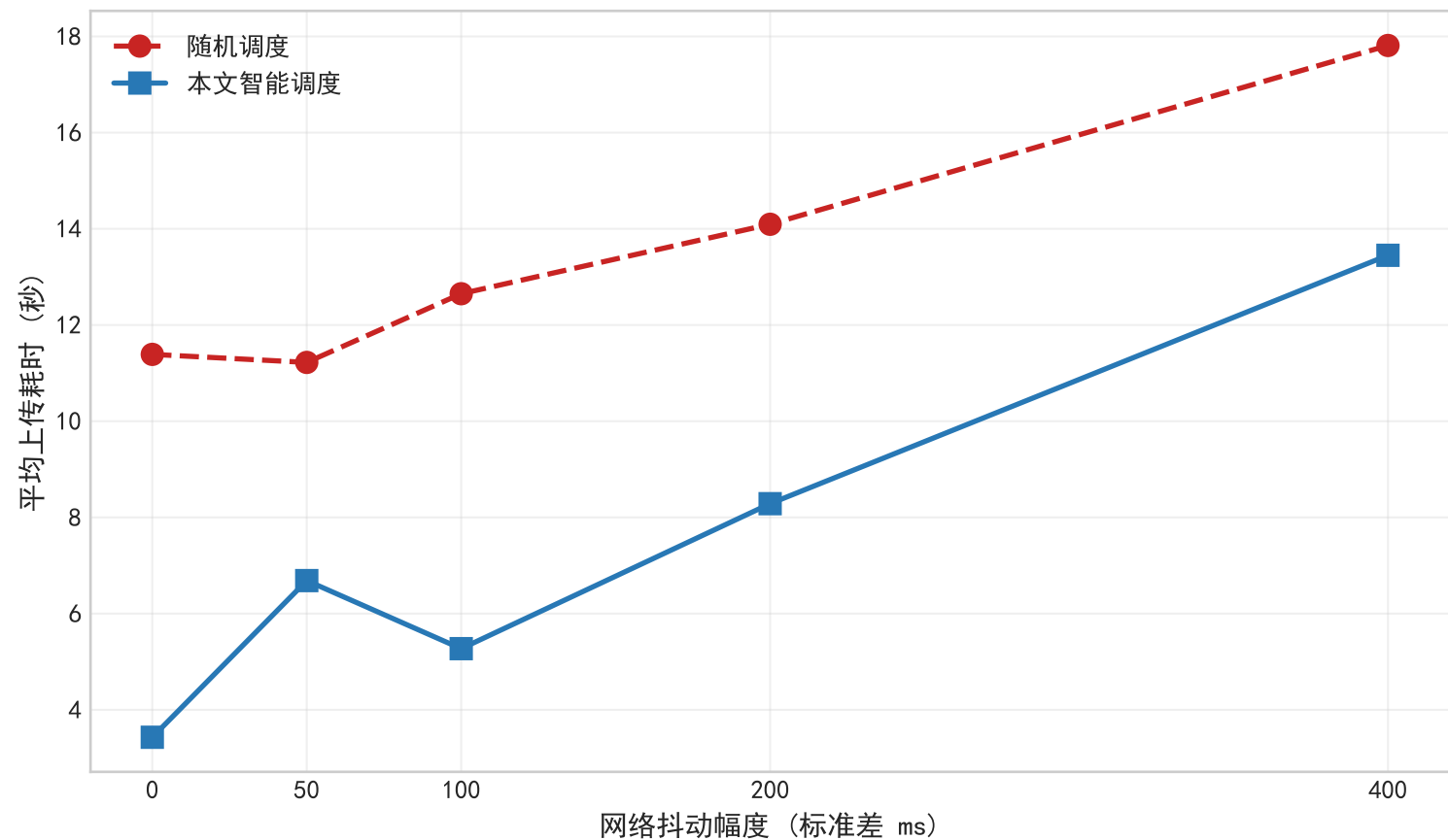
网络抖动对传输效率的影响
