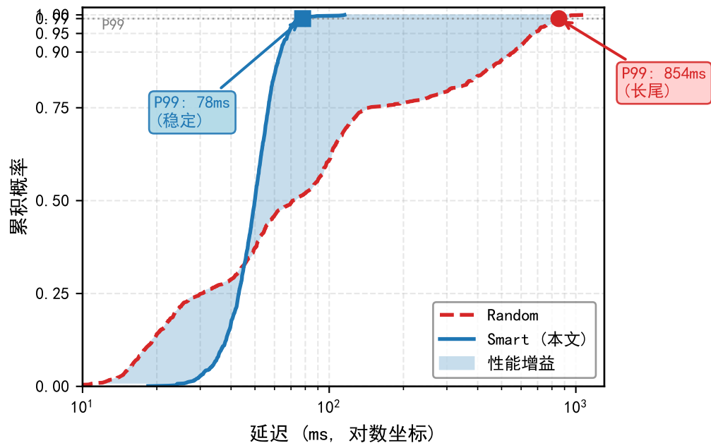
(b) 延迟分布 CDF (长尾消除)
