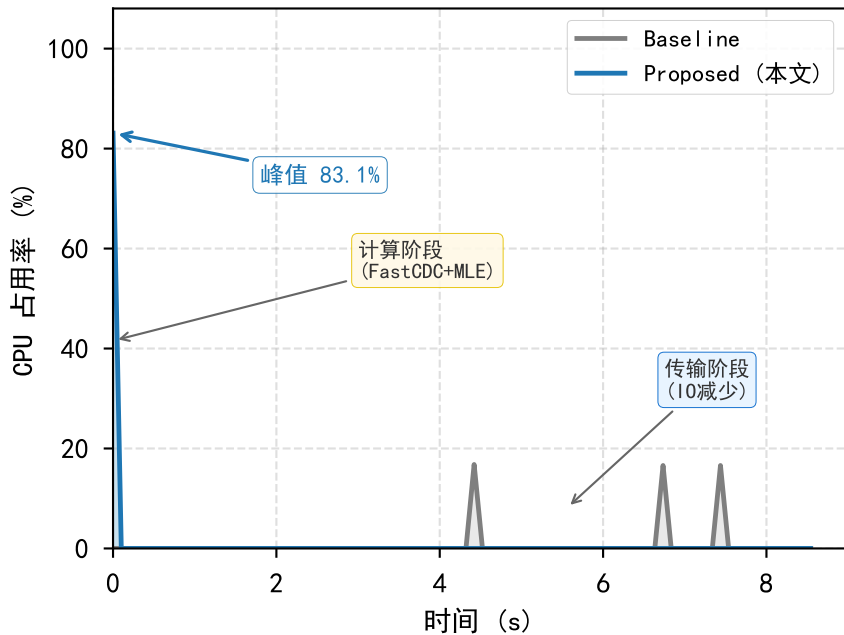
(a) CPU 占用率动态波形
