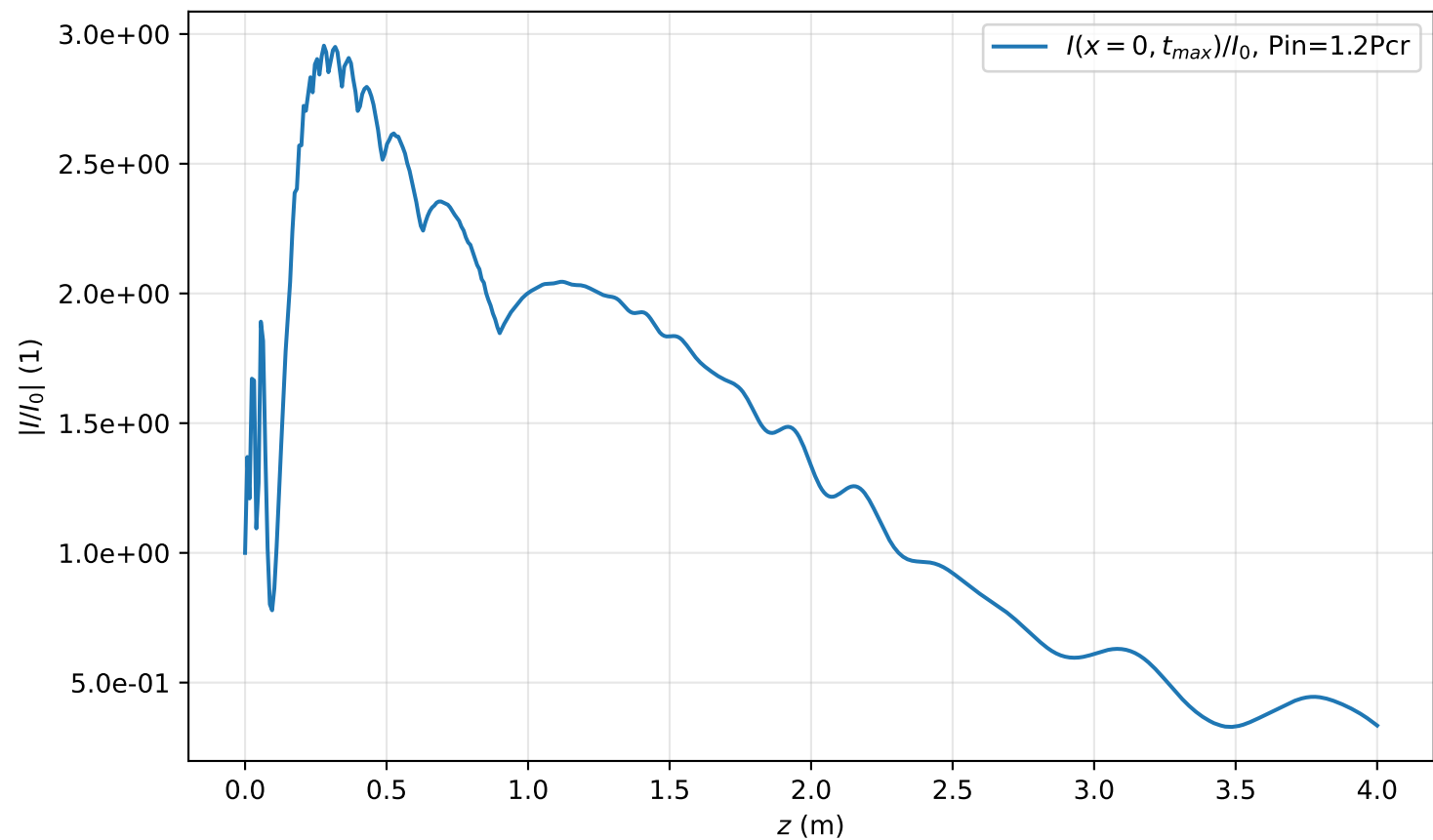
I(x=0, t_{max}, z)/I_0 , Pin=1.2Pcr
