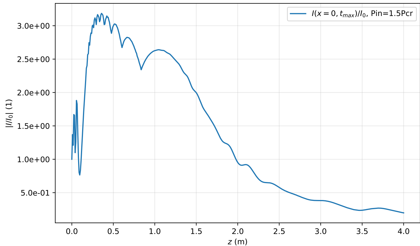
I(x=0, t_{max}, z)/I_0 , Pin=1.5Pcr
