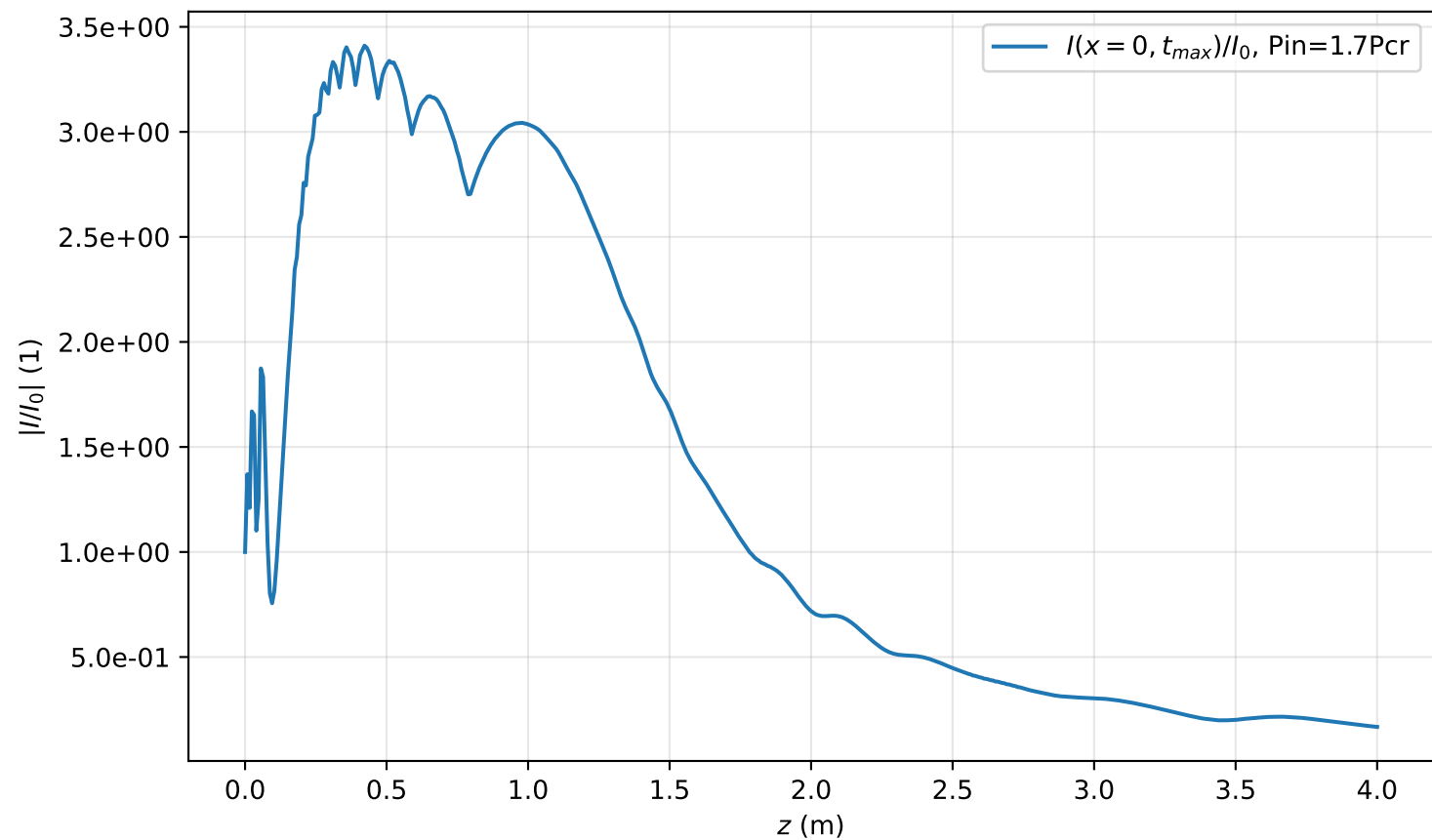
I(x=0, t_{max}, z)/I_0 , Pin=1.7Pcr
