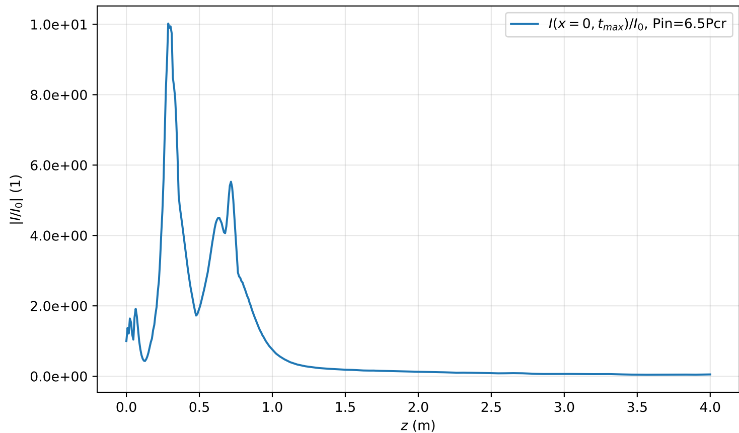
I(x=0, t_{max}, z)/I_0 , Pin=6.5Pcr
