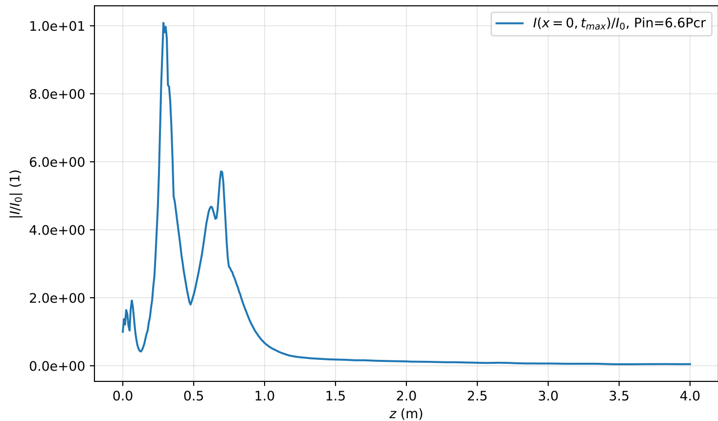
I(x=0, t_{max}, z)/I_0 , Pin=6.6Pcr
