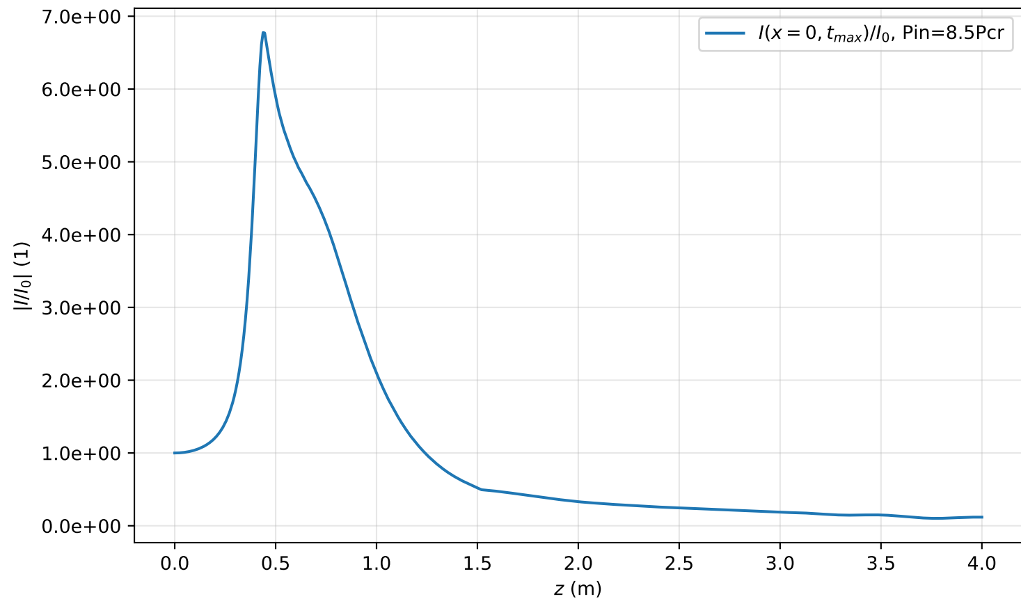
I(x=0, t_{max}, z)/I_0 , Pin=8.5Pcr
