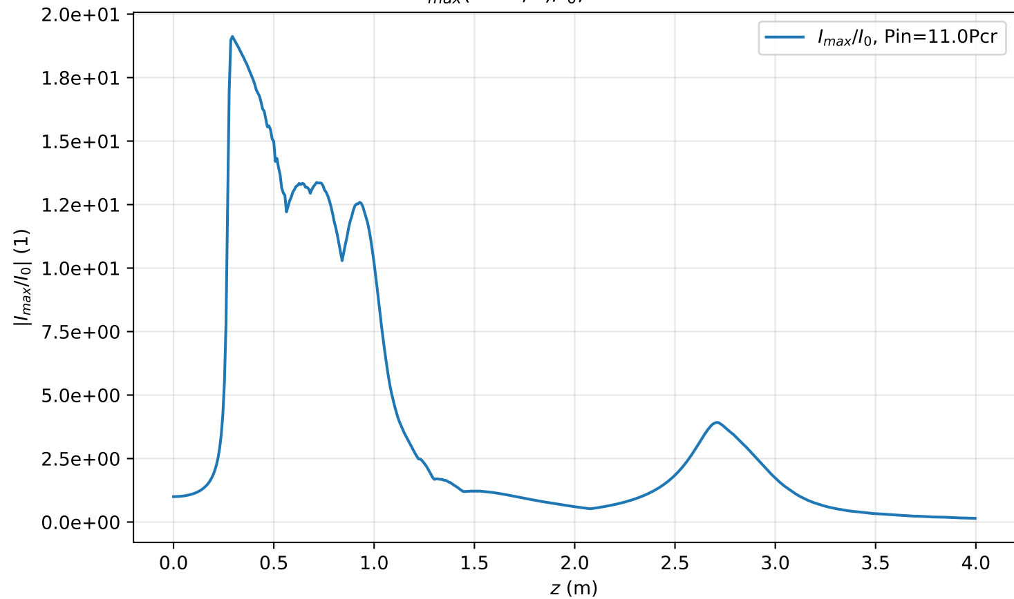
I_{max}(r=0, z)/I_0 , Pin=11.0Pcr
