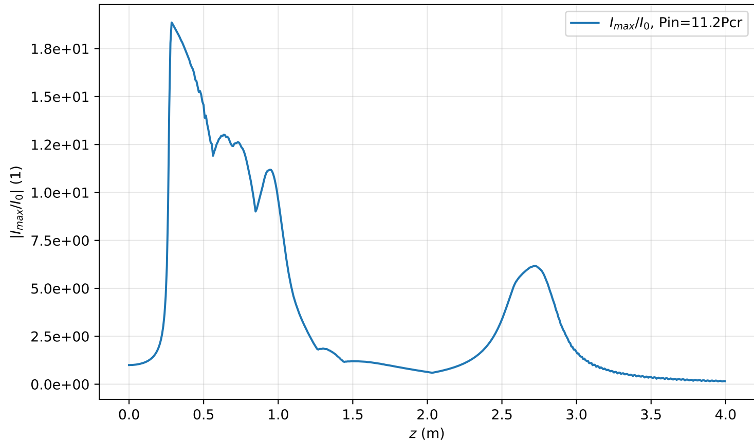
I_{max}(r=0, z)/I_0 , Pin=11.2Pcr
