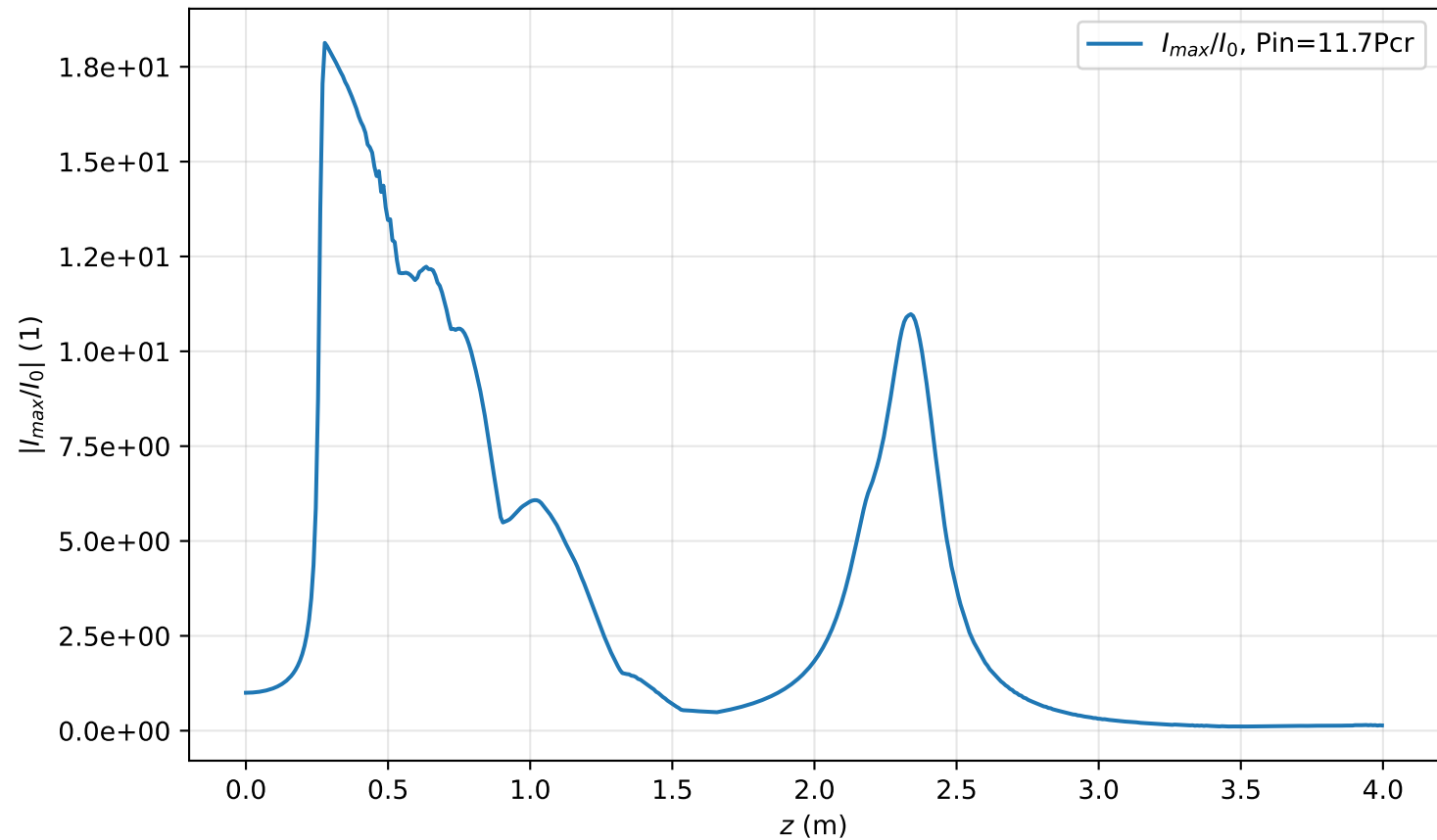
I_{max}(r=0, z)/I_0 , Pin=11.7Pcr
