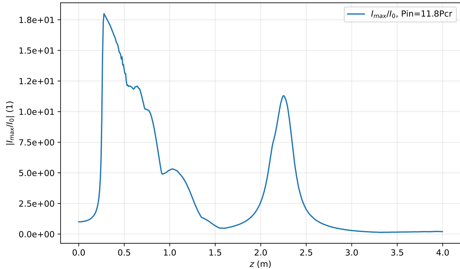
I_{max}(r=0, z)/I_0 , Pin=11.8Pcr
