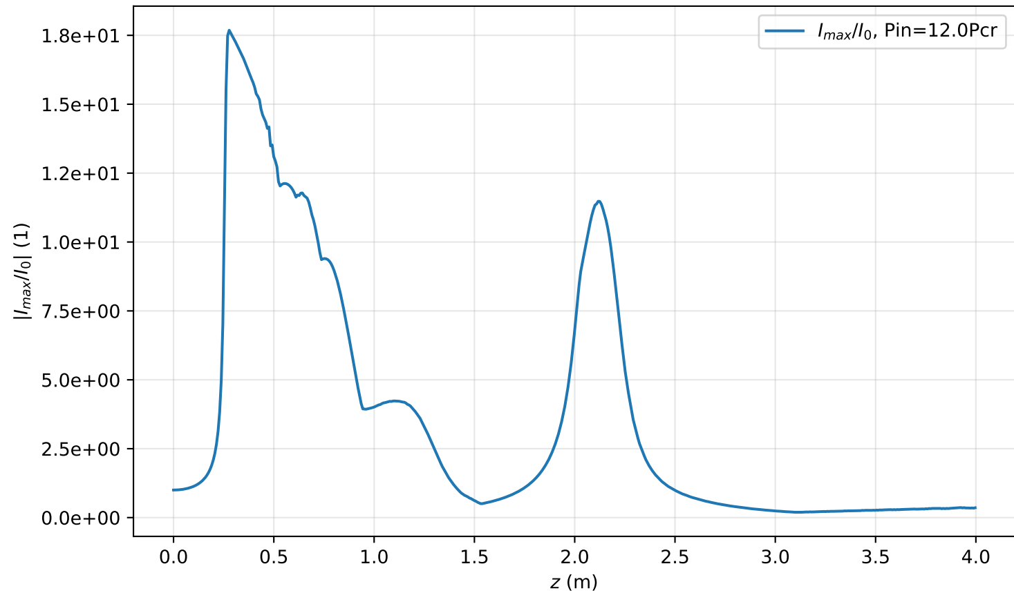
I_{max}(r=0, z)/I_0 , Pin=12.0Pcr
