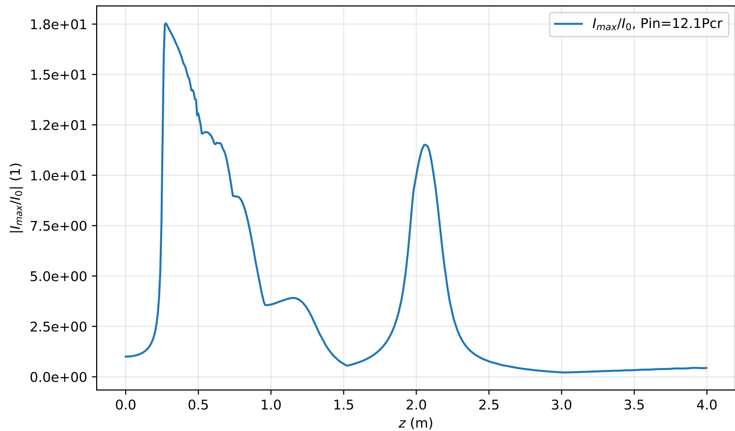
I_{max}(r=0, z)/I_0 , Pin=12.1Pcr
