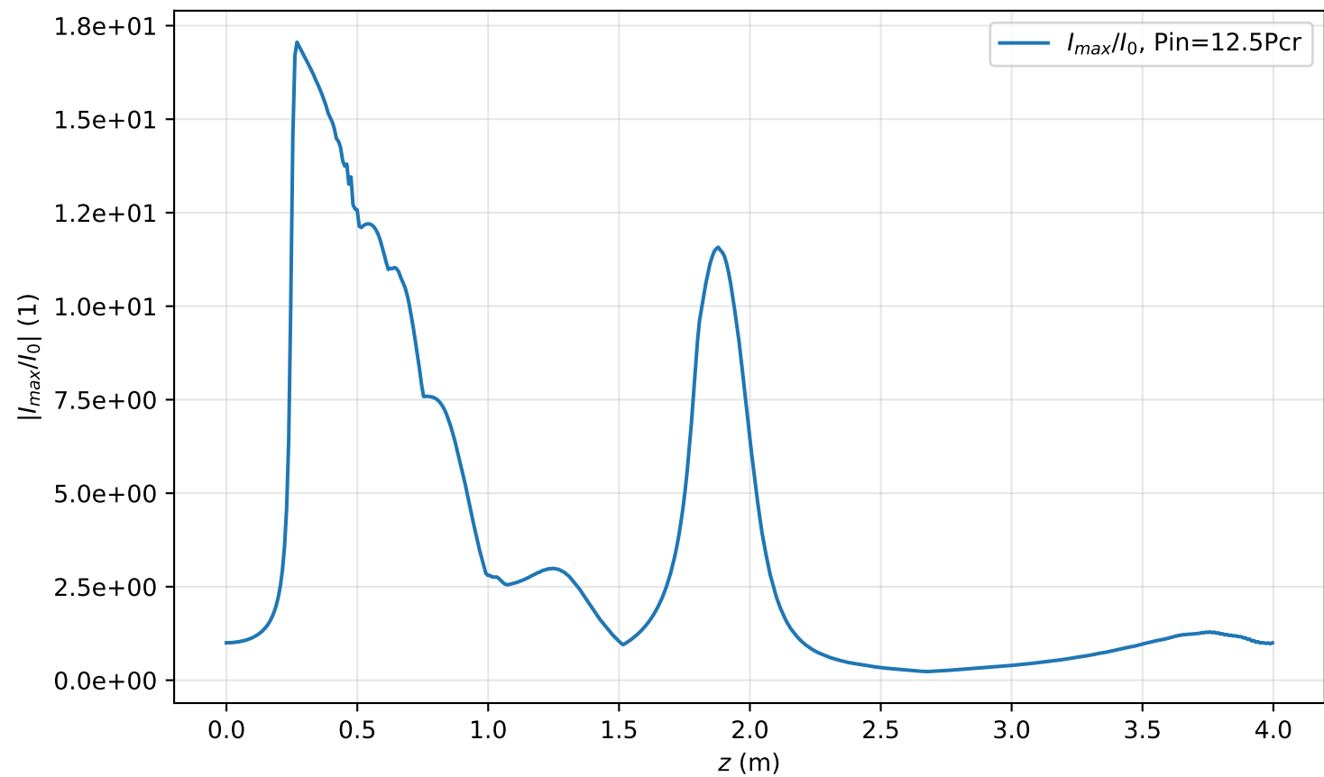
I_{max}(r=0, z)/I_0 , Pin=12.5Pcr
