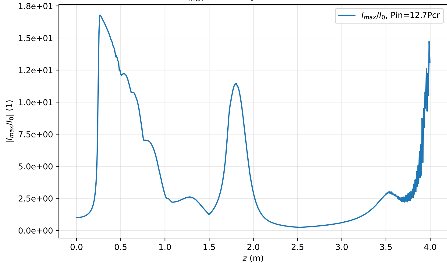
I_{max}(r=0, z)/I_0 , Pin=12.7Pcr
