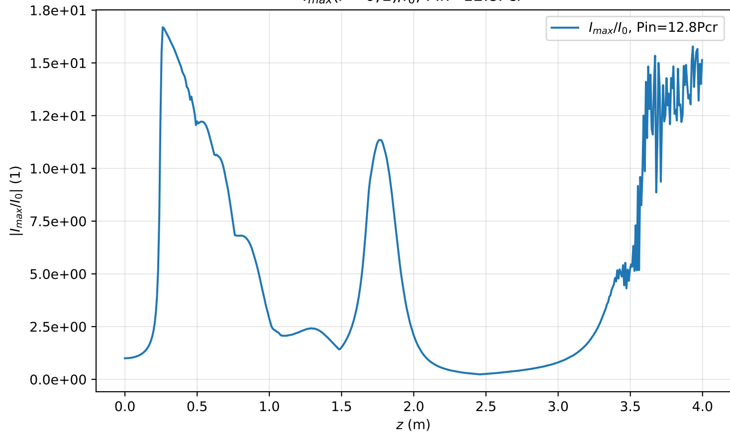
I_{max}(r=0, z)/I_0 , Pin=12.8Pcr
