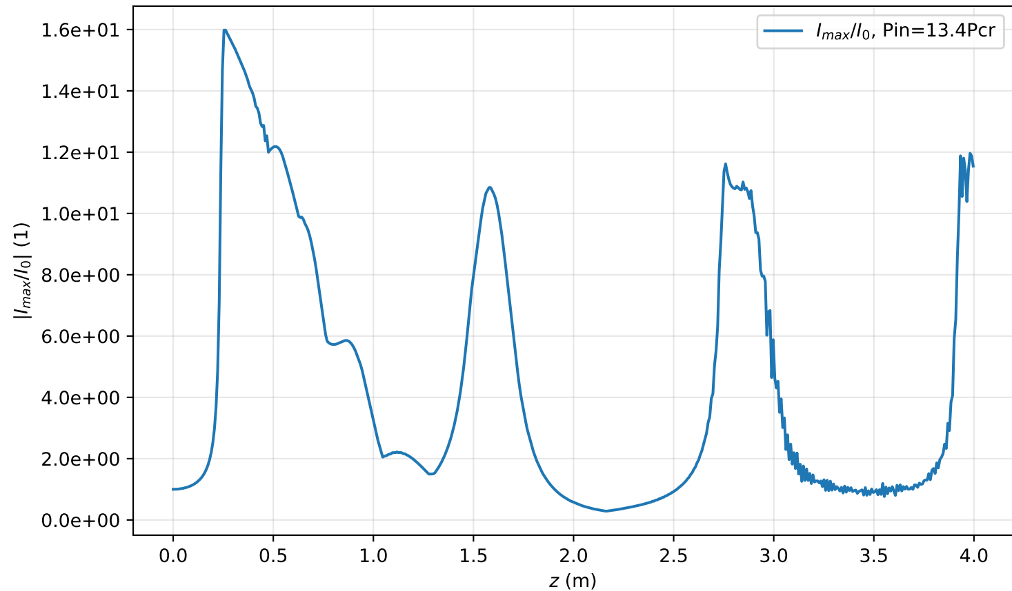
I_{max}(r=0, z)/I_0 , Pin=13.4Pcr
