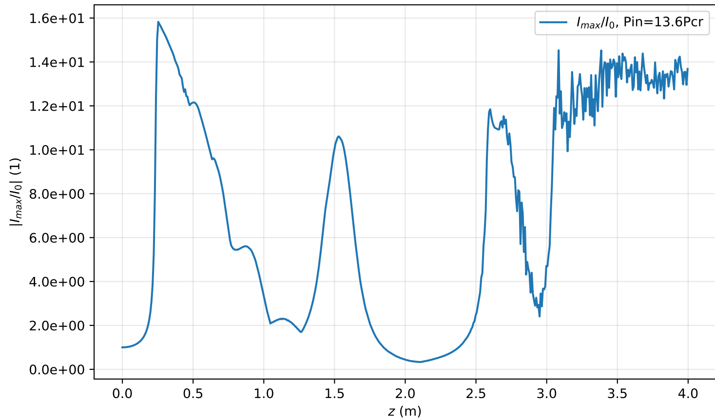
I_{\max}(r=0, z)/I_0 , Pin=13.6Pcr
