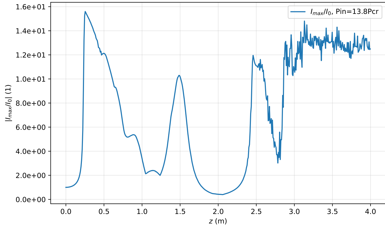
I_{\max}(r=0, z)/I_0 , Pin=13.8Pcr
