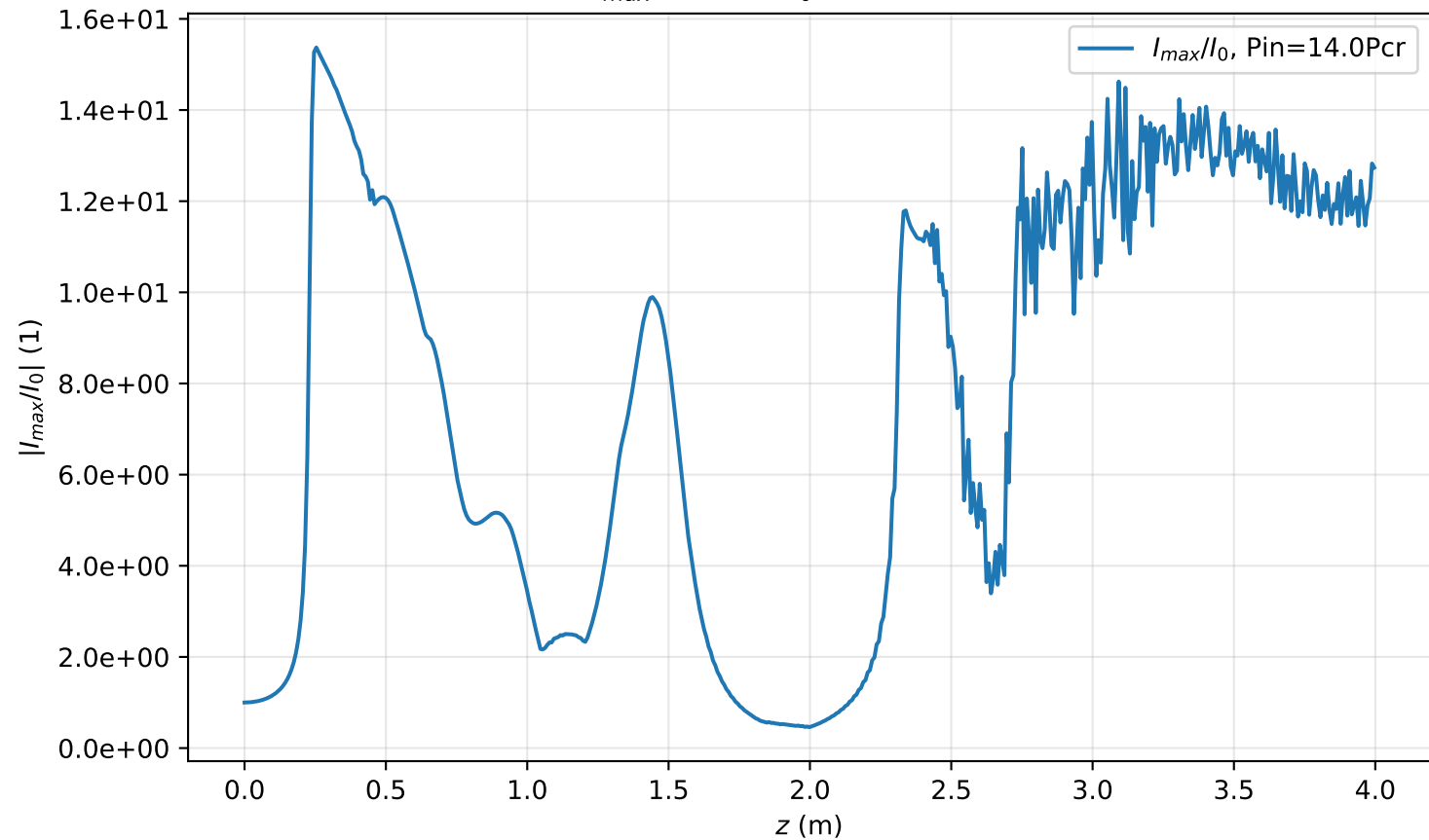
I_{\max}(r=0, z)/I_0 , Pin=14.0Pcr
