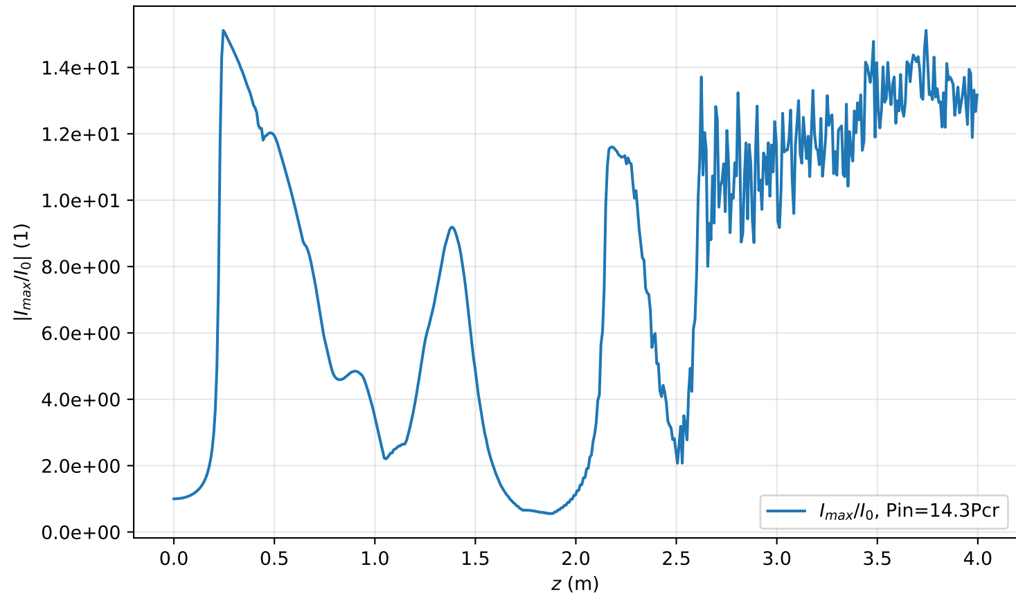
I_{\max}(r=0, z)/I_0 , Pin=14.3Pcr
