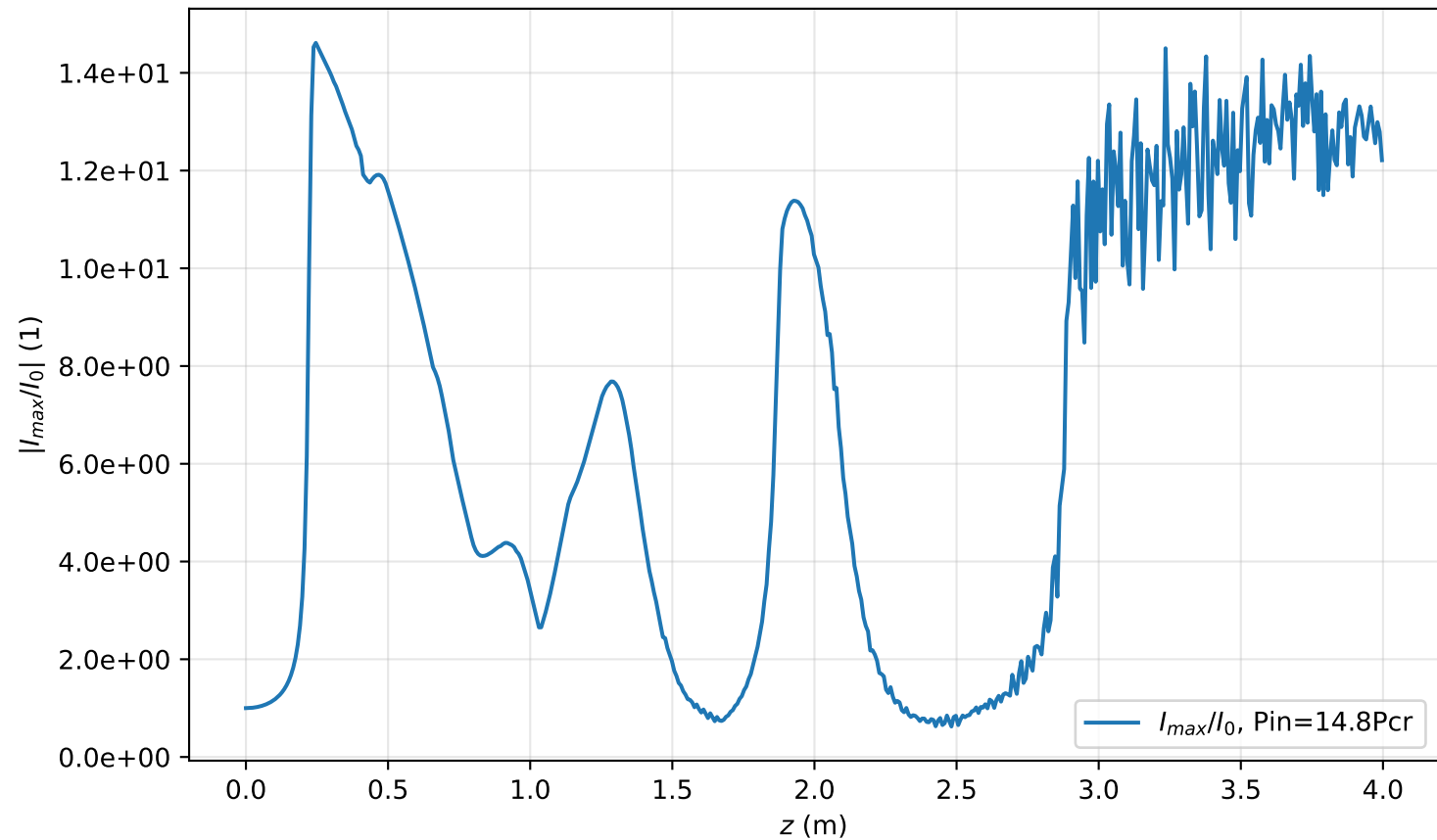
I_{max}(r=0, z)/I_0 , Pin=14.8Pcr
