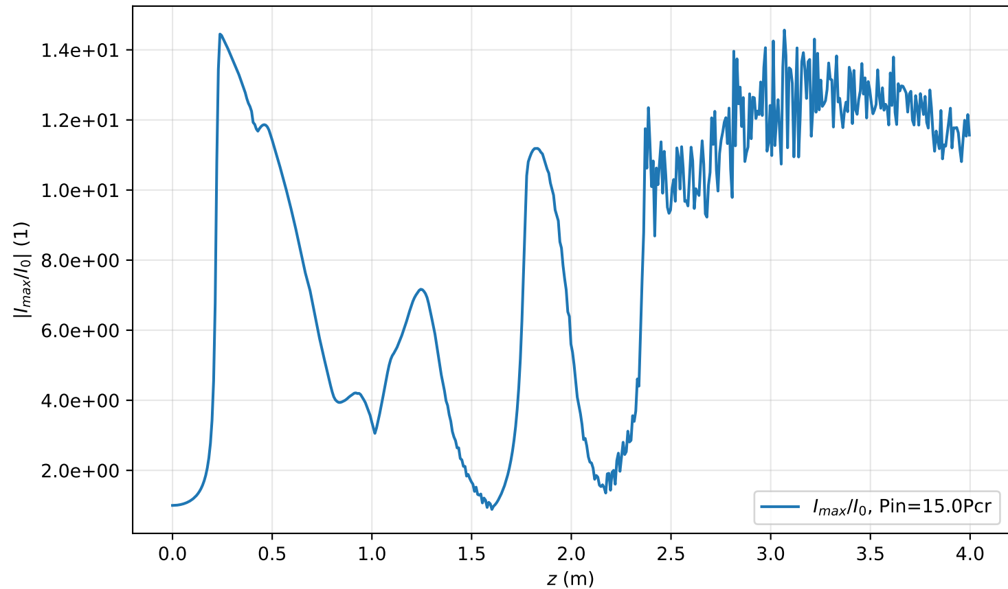
I_{max}(r=0, z)/I_0 , Pin=15.0Pcr
