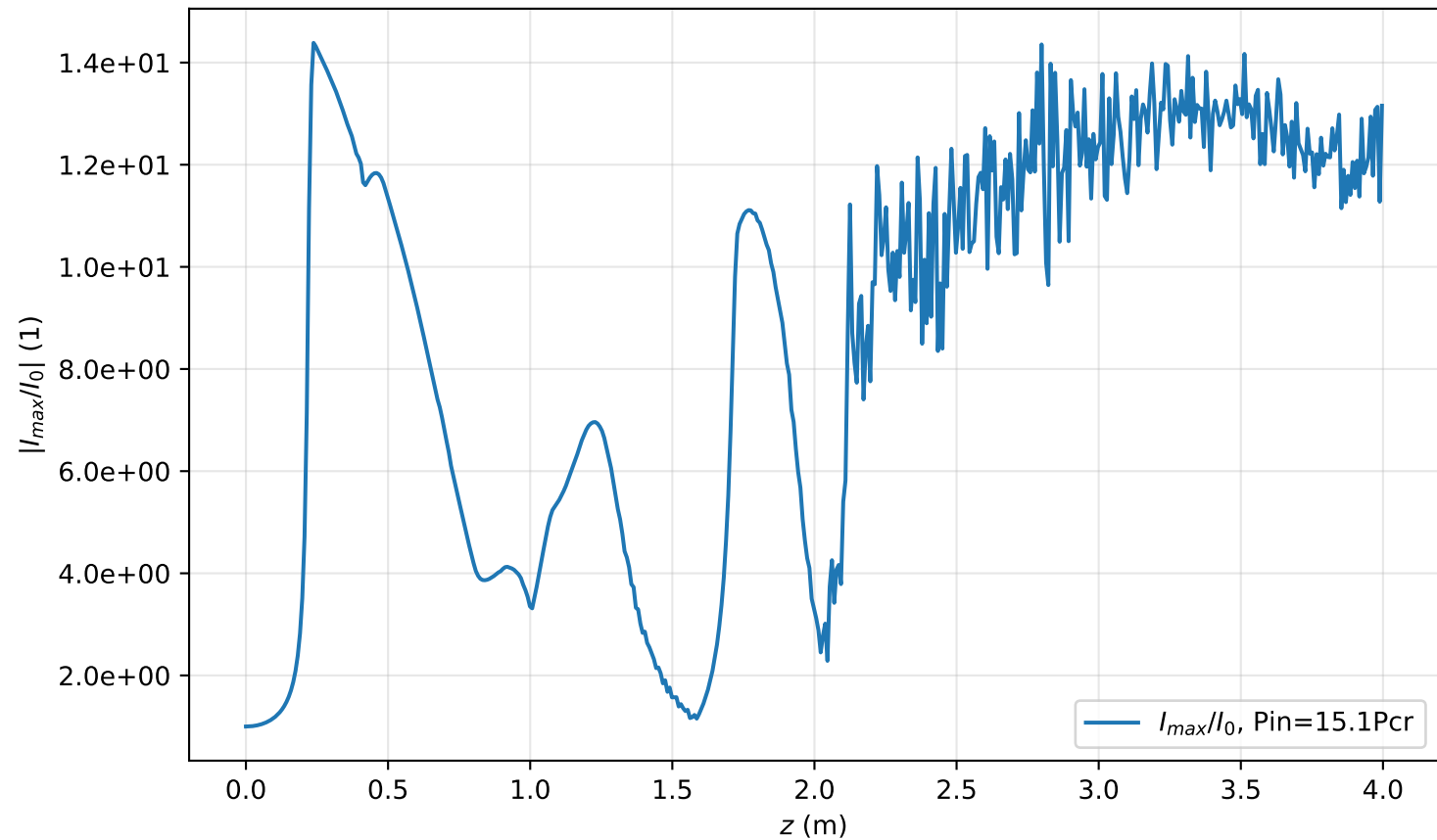
I_{max}(r=0, z)/I_0 , Pin=15.1Pcr
