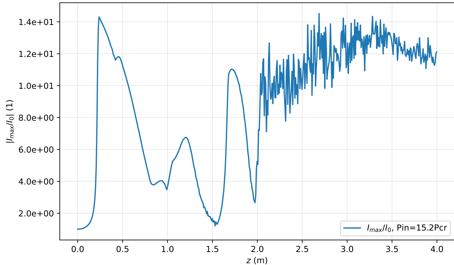
I_{max}(r=0, z)/I_0 , Pin=15.2Pcr
