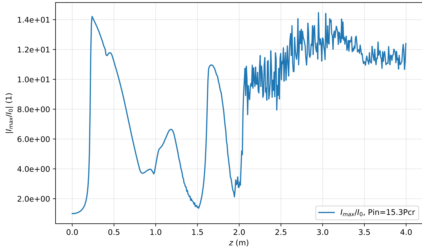
I_{max}(r=0, z)/I_0 , Pin=15.3Pcr
