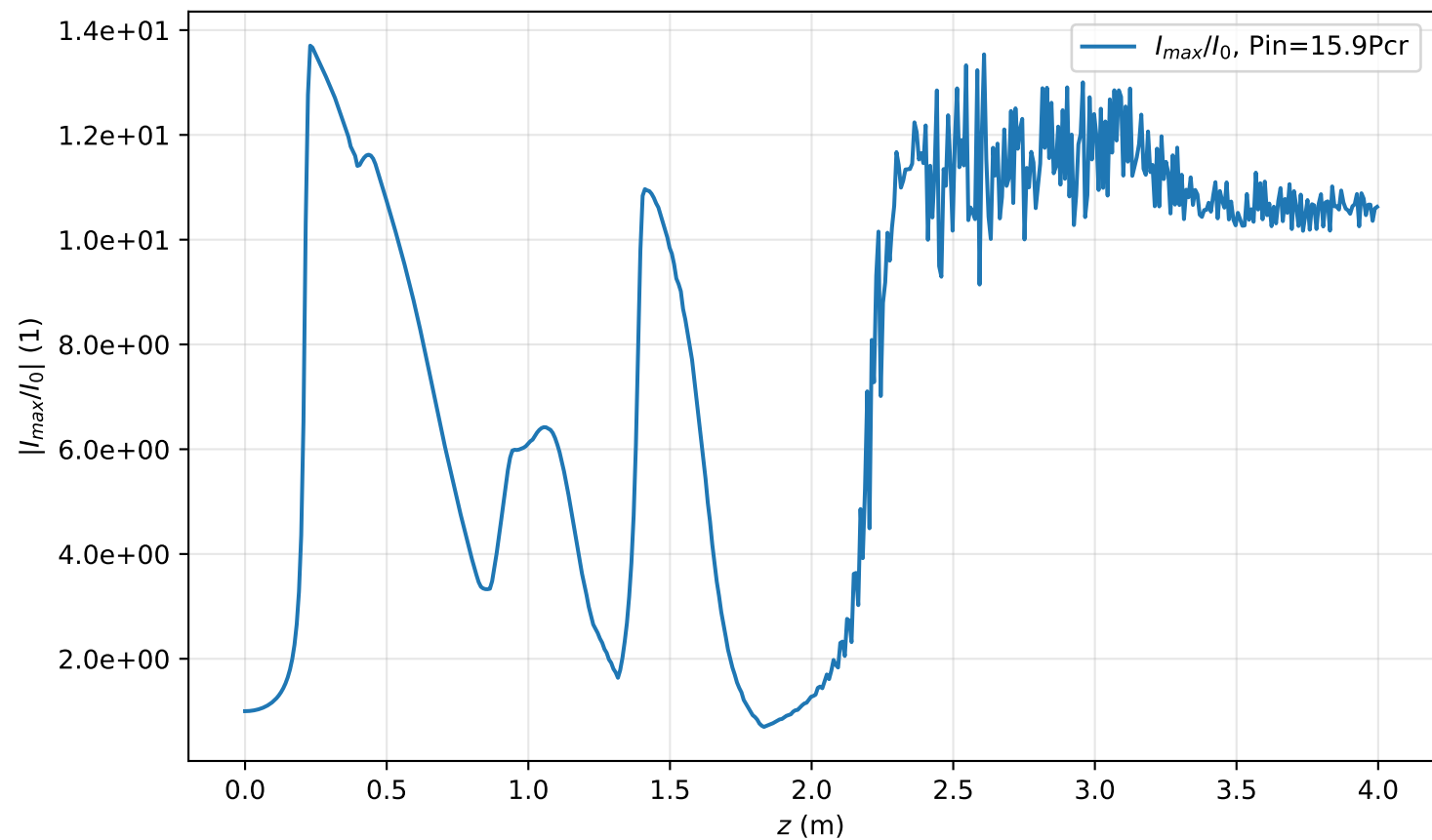
I_{\max}(r=0, z)/I_0 , Pin=15.9Pcr
